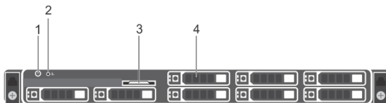
図 3. ホットスワップ対応 2.5 インチハードドライブ 8 台搭載シャーシの前面パネル機能
