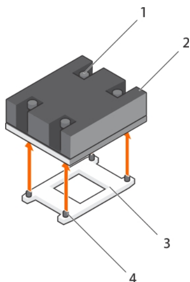
図 41. ヒートシンクの取り外し
