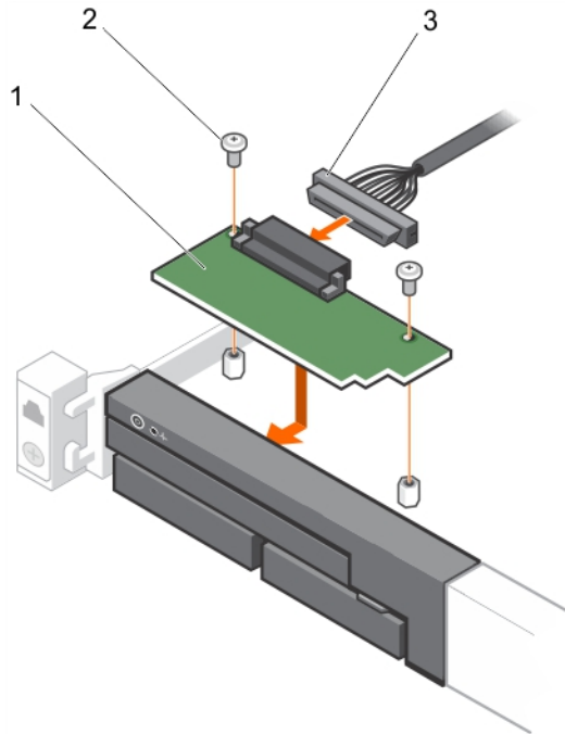
図 68. コントロールパネルモジュールの取り付け - ハードドライブ 8 台搭載シャーシ
