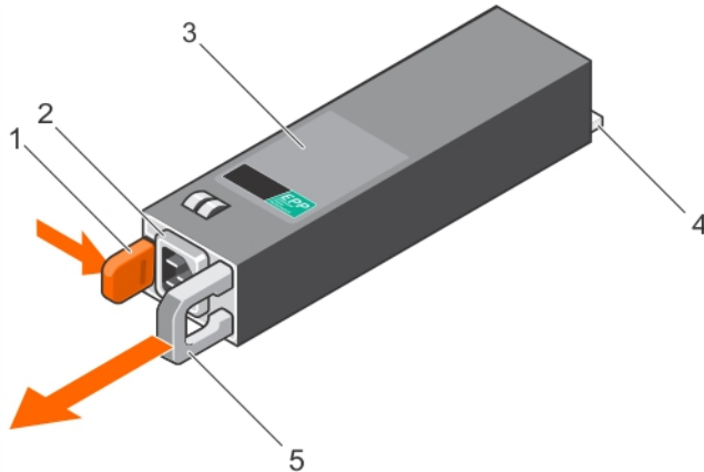
図 47. 冗長 PSU の取り外し
