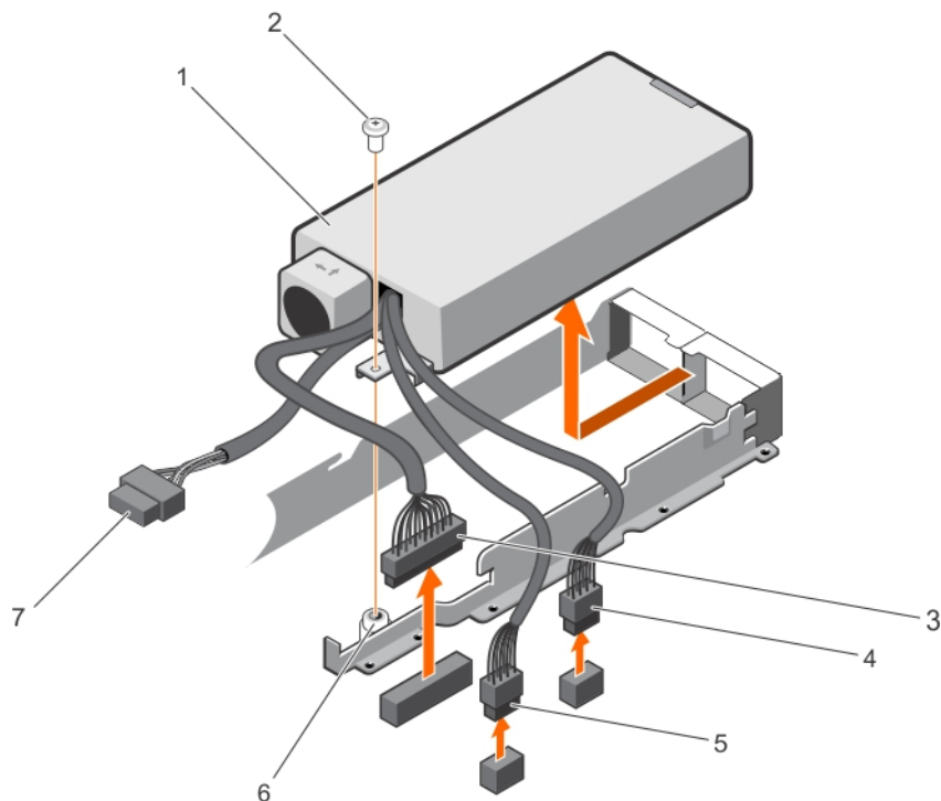
図 49. ケーブル接続式 PSU の取り付け
