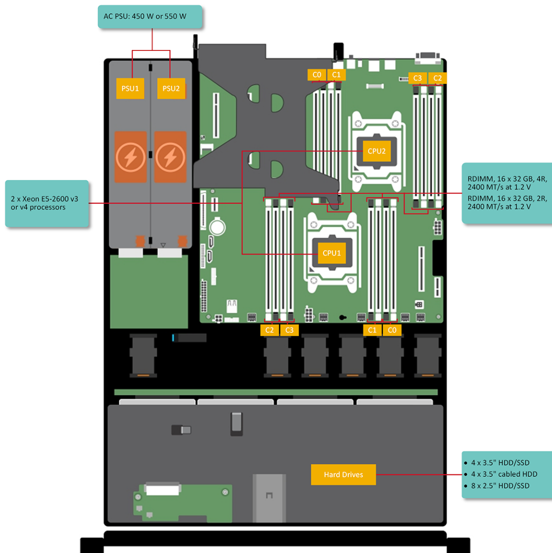
図 1. サポートされている構成のシステム表示
