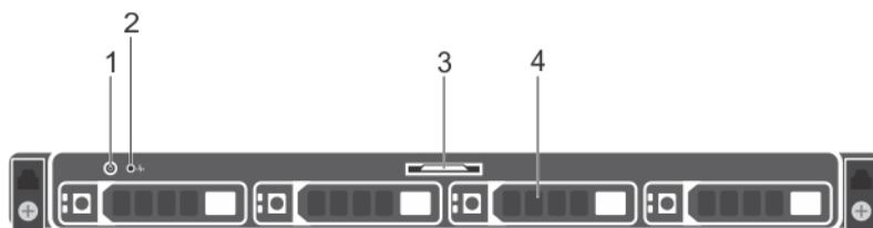
図 2. ホットスワップ対応 3.5 インチハードドライブ 4 台搭載シャーシの前面パネル機能
