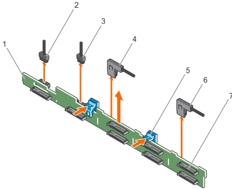
図 57. 2.5 インチハードドライブ 8 台搭載の SAS/SATA バックプレーンの取り外し
