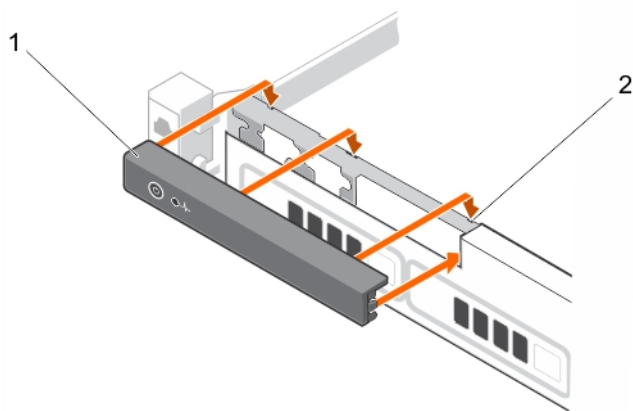
図 63. コントロールパネルの取り付け - 3.5 インチハードドライブ 4 台搭載シャーシ
