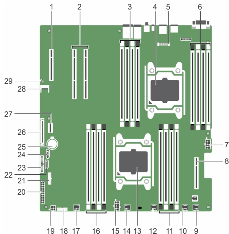
図 75. システム基板のジャンパとコネクタ
