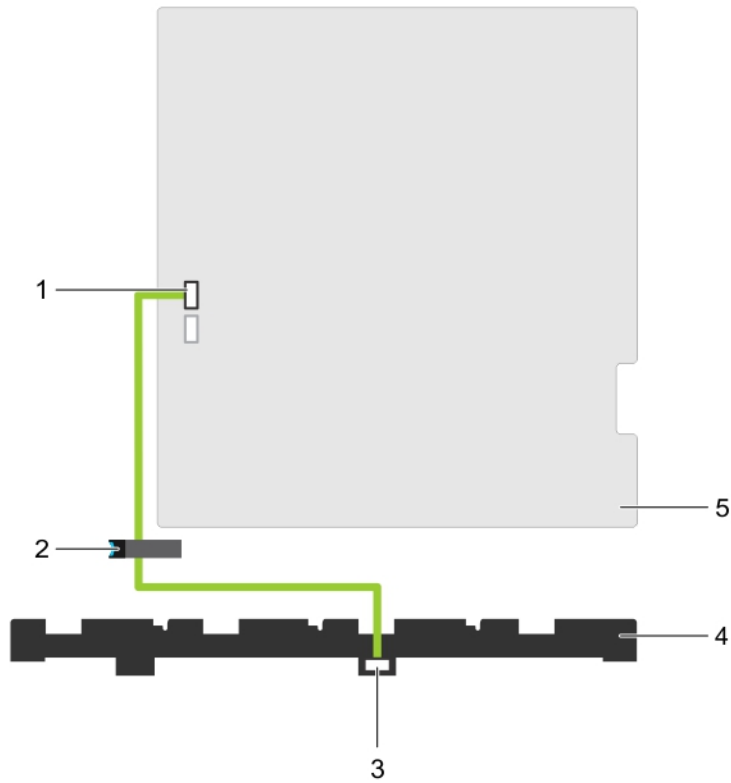
図 56. ケーブル配線図 - 3.5 インチ 4 台搭載 (x4) の SAS/SATA バックプレーン
