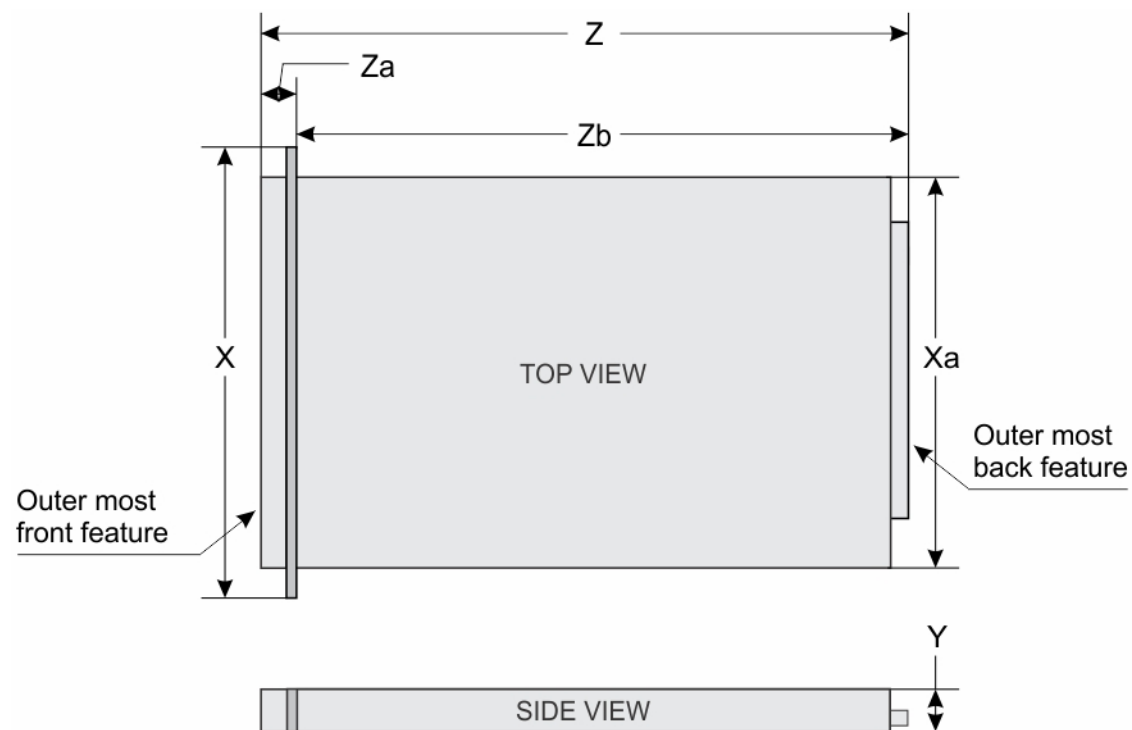
図 11. Dell DSS 1500 システムのシャーシ寸法
