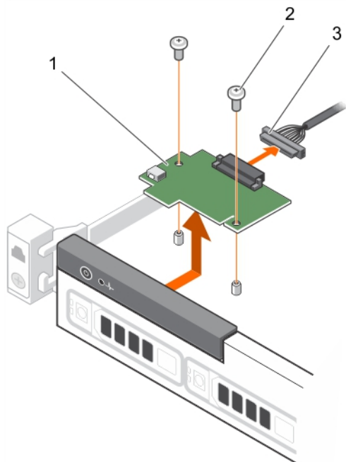
図 65. コントロールパネルモジュールの取り外し - ハードドライブ 4 台搭載シャーシ
