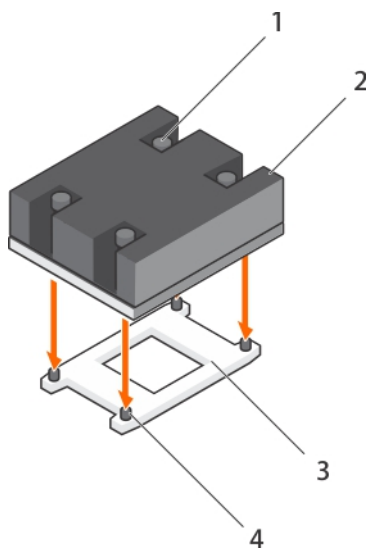
図 46. ヒートシンクの取り付け
