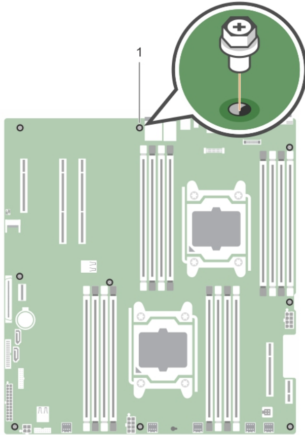
図 71. システム基板上のネジの位置
