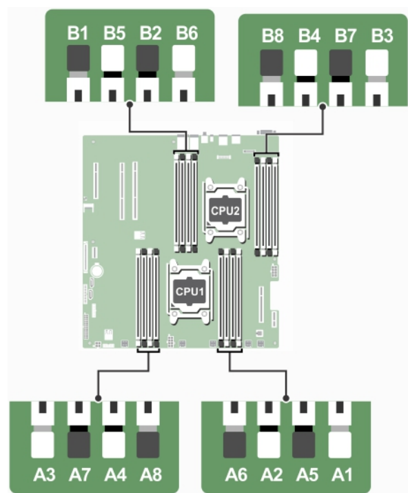
図 18. メモリソケットの位置
