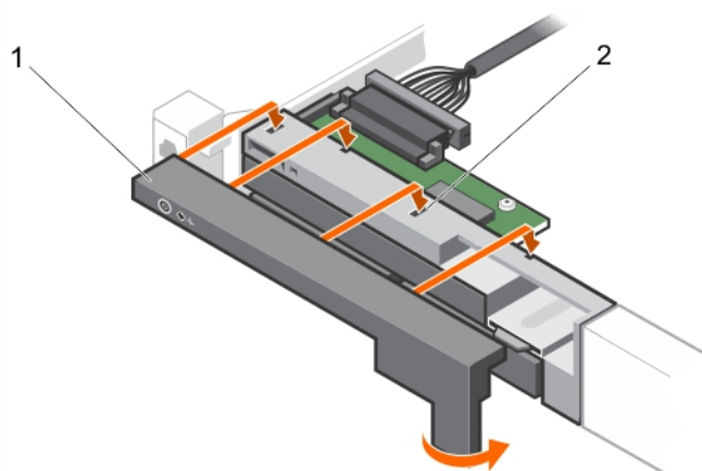
図 64. コントロールパネルの取り付け - 2.5 インチハードドライブ 8 台搭載シャーシ
