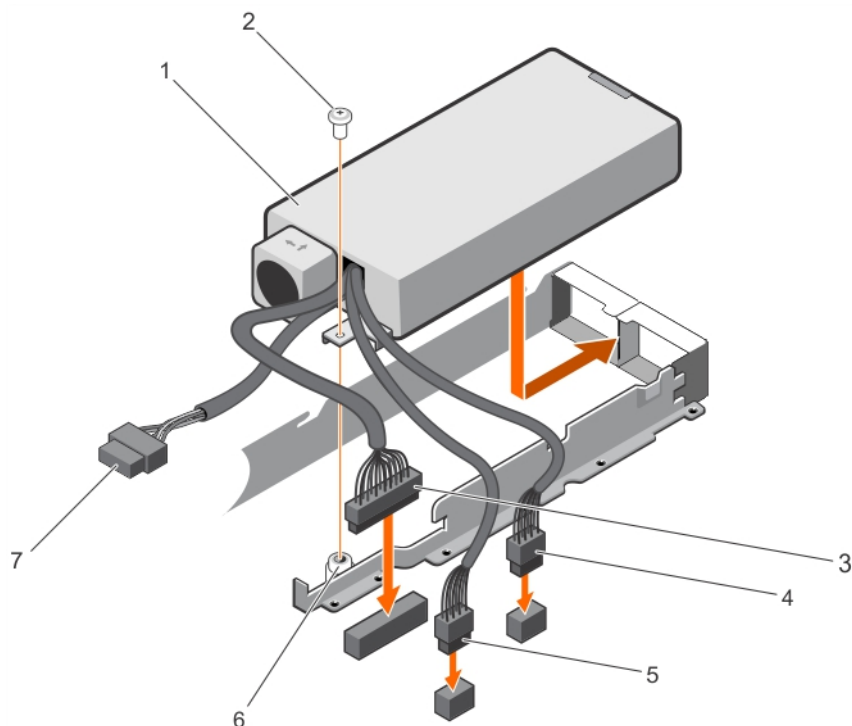
図 50. 非冗長 PSU の取り付け
