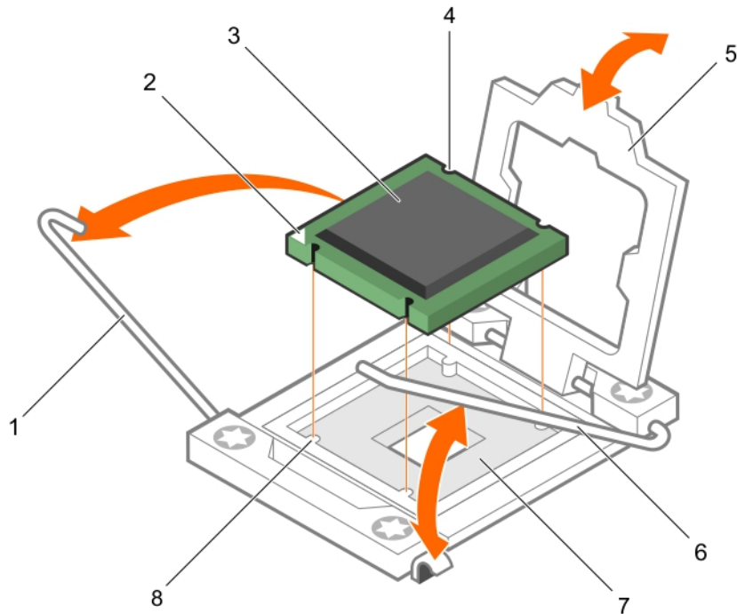
図 44. プロセッサの取り付け
