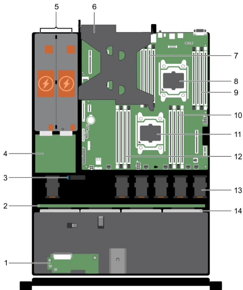
図 15. システムの内部 - 冗長電源装置搭載
