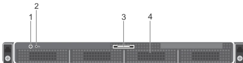
図 4.3.5 インチハードドライブ 4 台搭載シャーシの前面パネル機能
