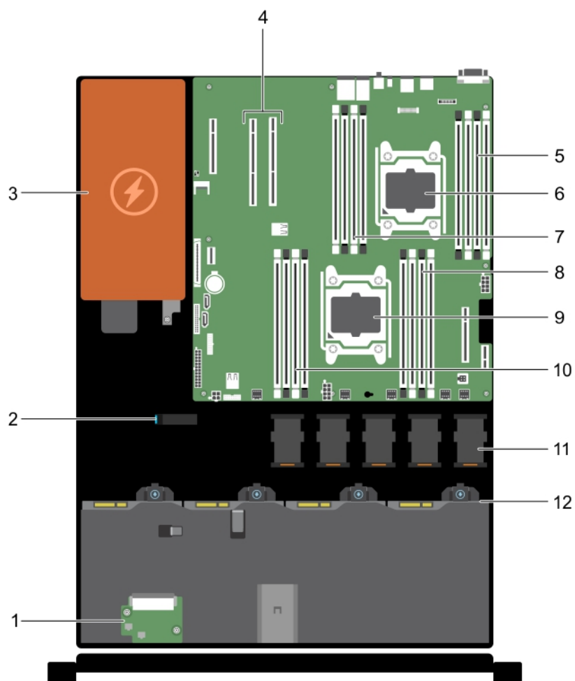
図 14. システムの内部 – 非冗長電源装置搭載
