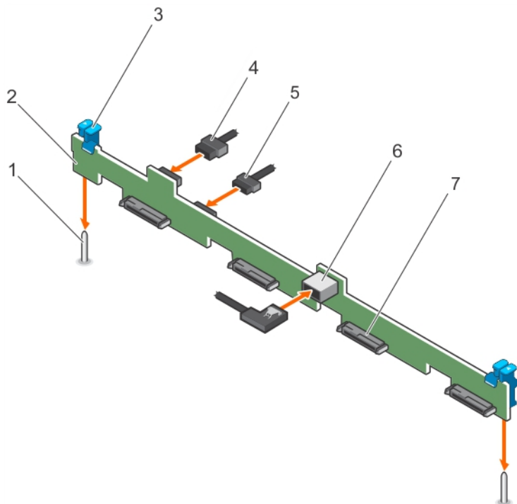
図 59. 3.5 インチハードドライブ 4 台搭載の SAS/SATA バックプレーンの取り付け
