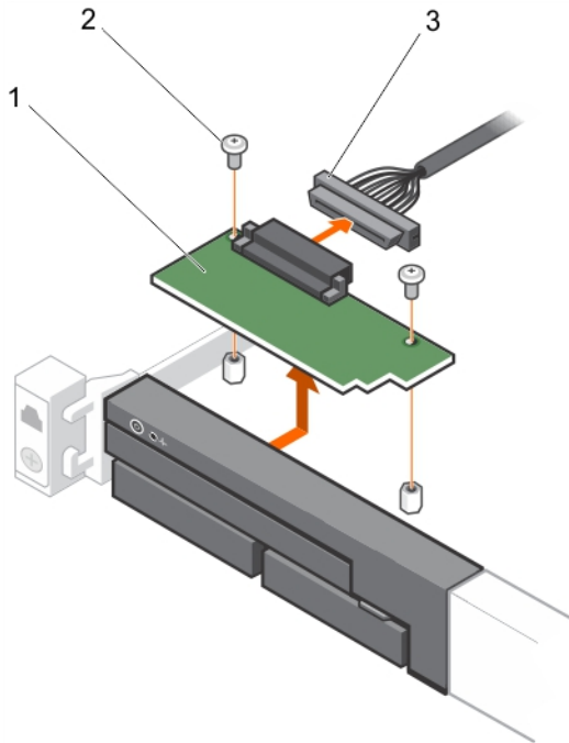
図 66. コントロールパネルモジュールの取り外し - ハードドライブ 8 台搭載シャーシ
