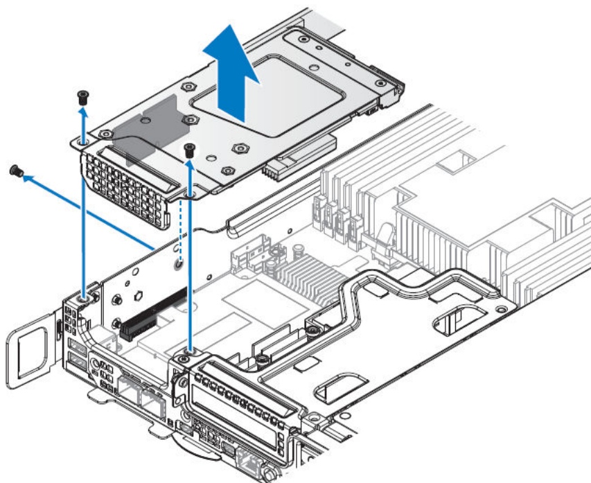
図 66. Mini PERC アセンブリの取り外し
