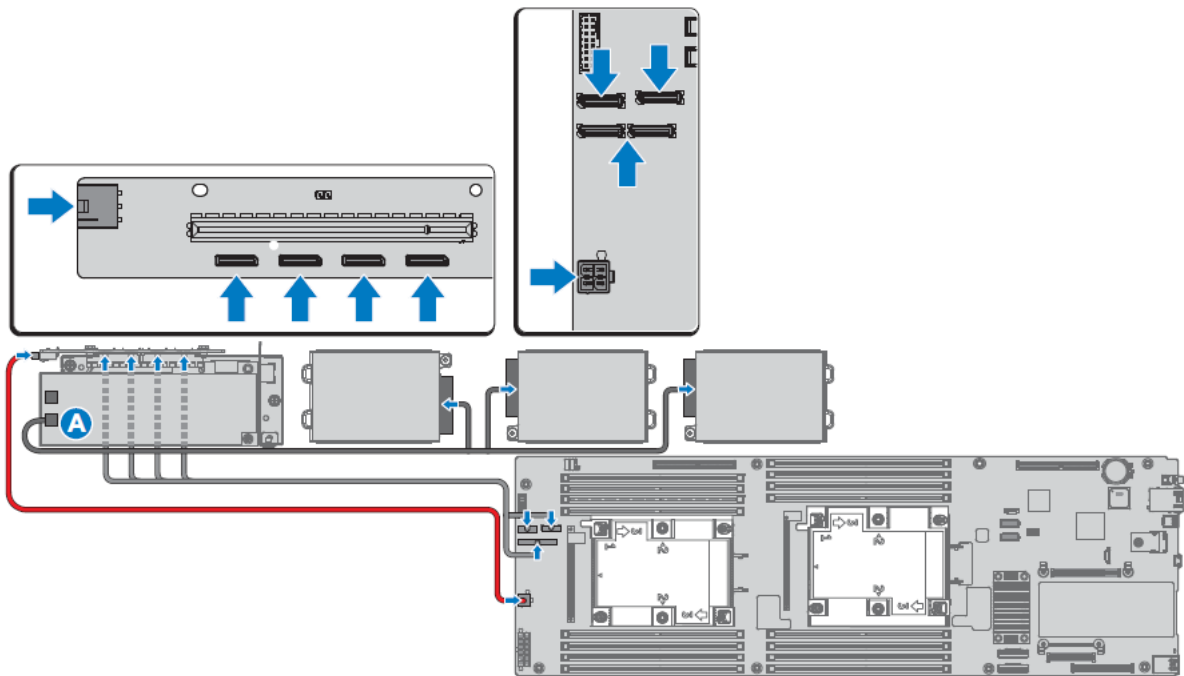
図 135. ケーブルの接続
