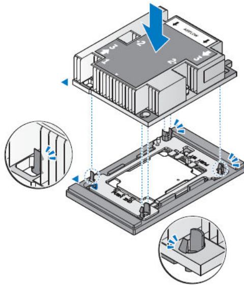
図 19. プロセッサトレイアセンブリへのヒートシンクの挿入
