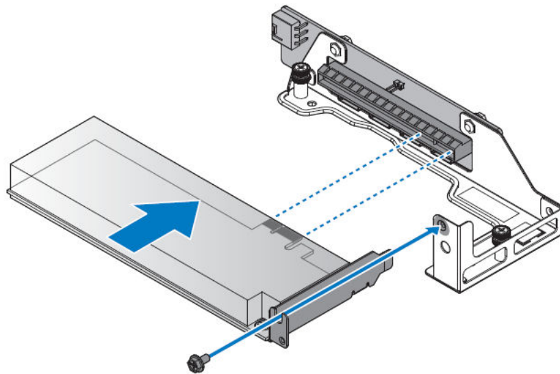
図 133. ブラケットへの NPIO カードの取り付け
