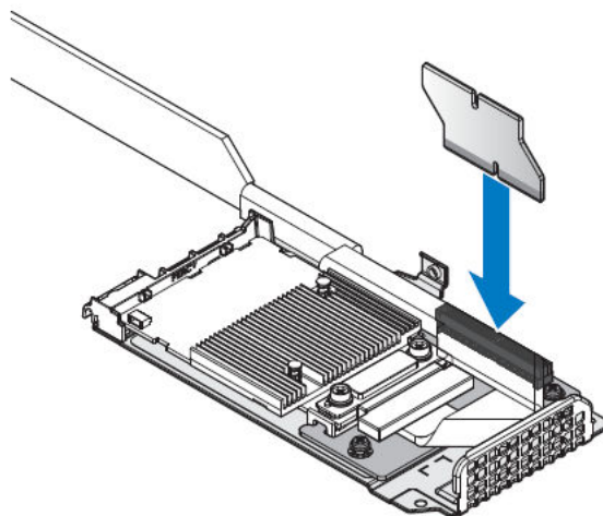
図 72. Mini PERC アセンブリへのブリッジボードの取り付け
