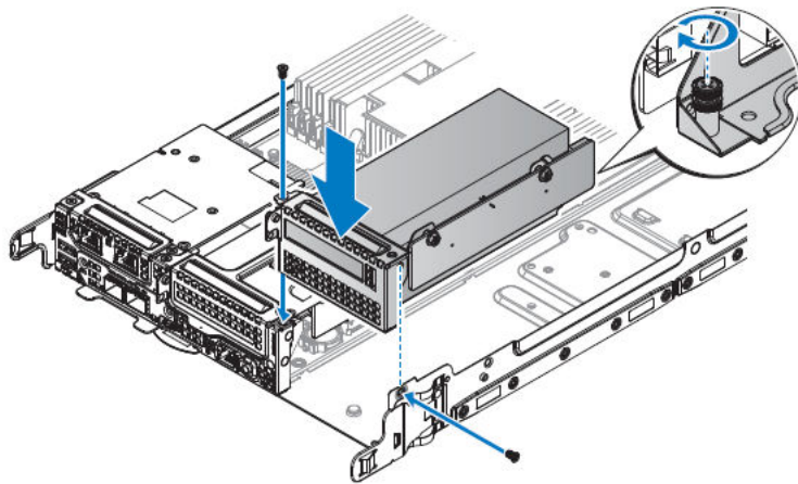
図 141. NPIO カードアセンブリの取り付け
