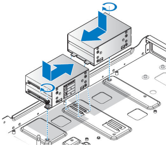
図 31. 2.5 インチ HDD アセンブリの取り付け
