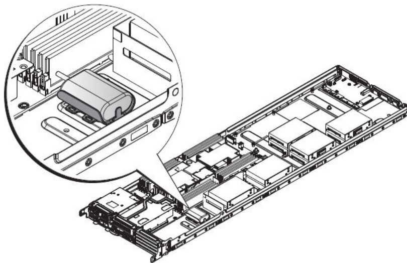
図 52. スーパーキャパシタの位置の確認
