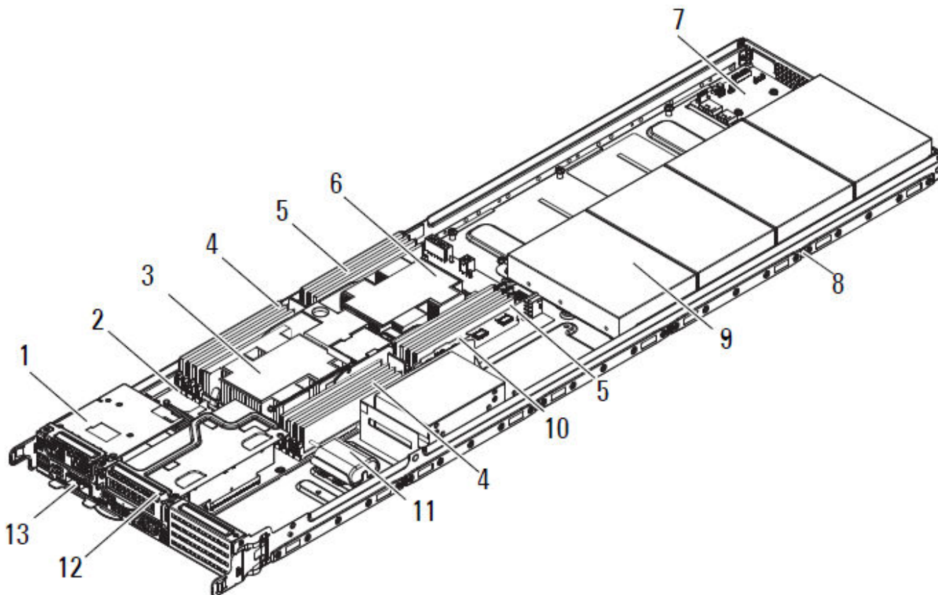
図 2. DSS 9620 3.5 インチハーフワイドサーバ
