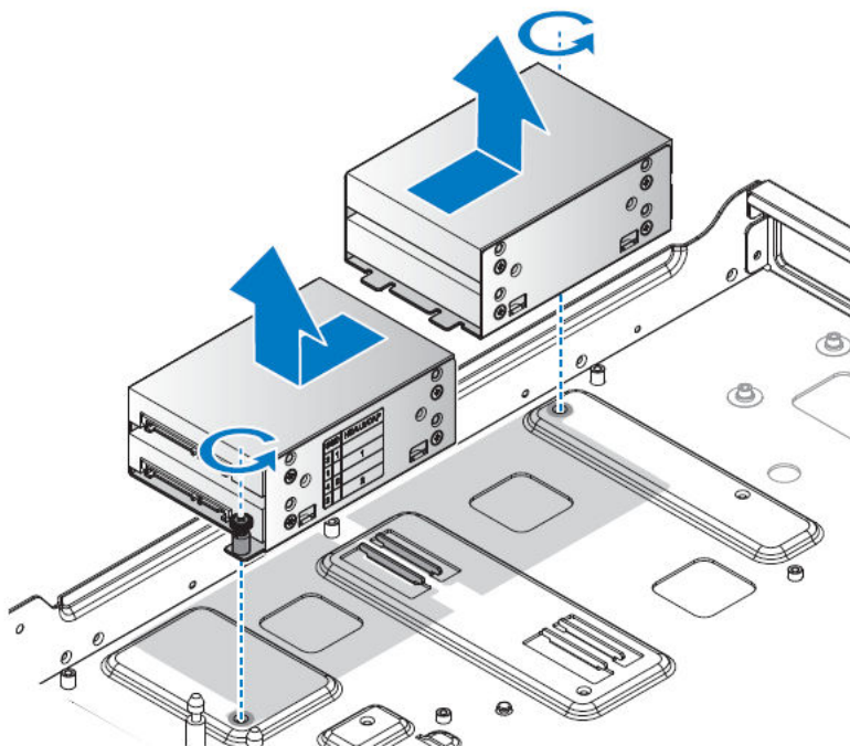
図 28. 2.5 インチ HDD アセンブリの取り外し
