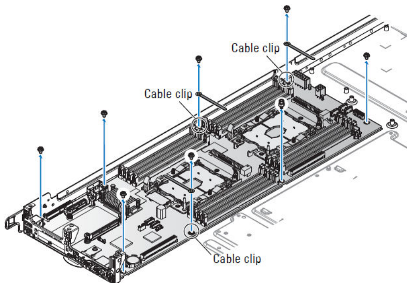
図 42. サーバボードの固定ネジの取り外し
