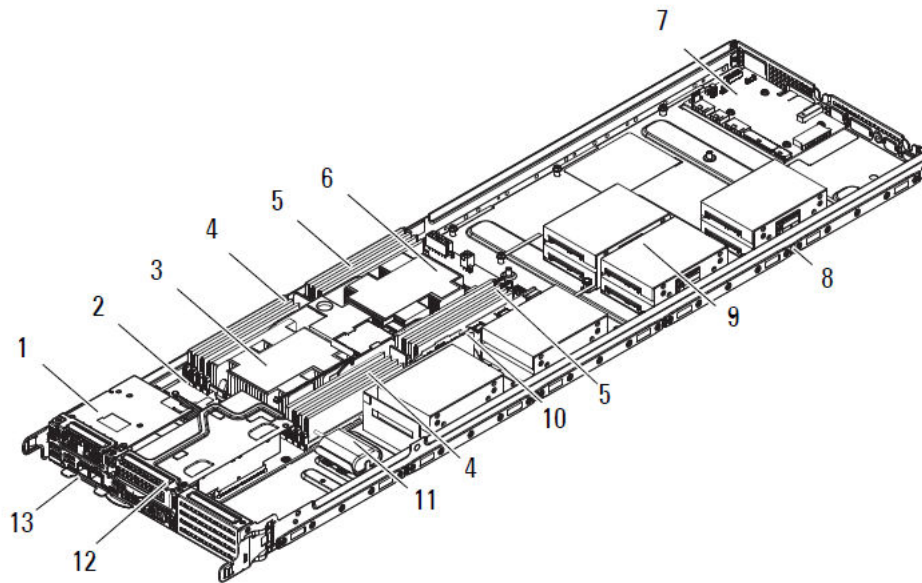
図 1. DSS 9620 2.5 インチーフワイドサーバ
