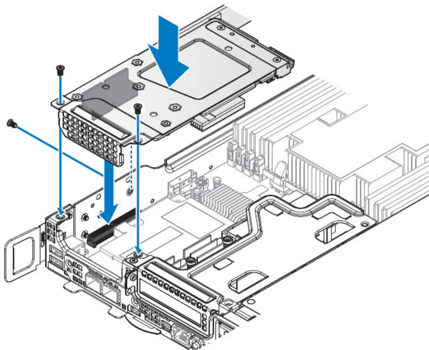
図 73. Mini PERC アセンブリの取り付け
