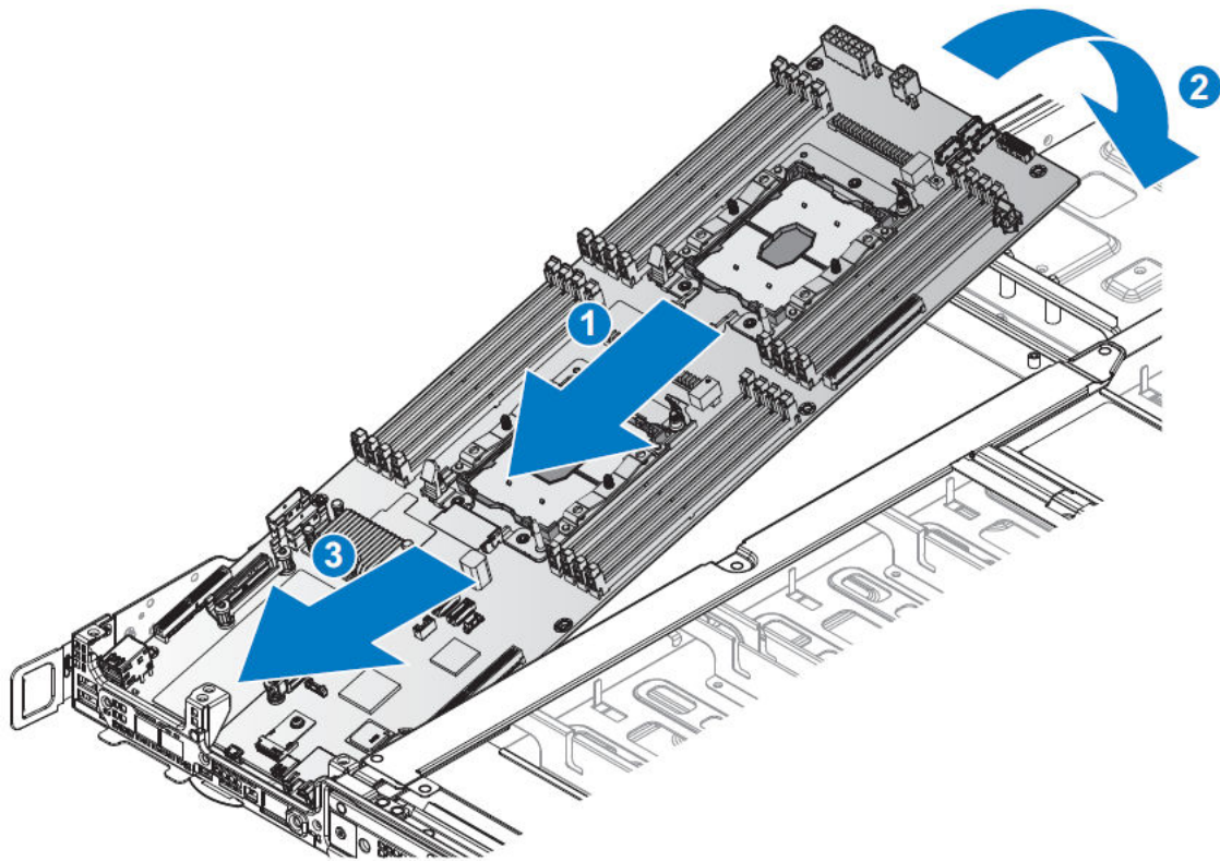
그림 44. 서버 보드 설치
