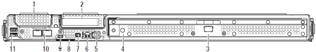
그림 3. 전면 패널 구조
