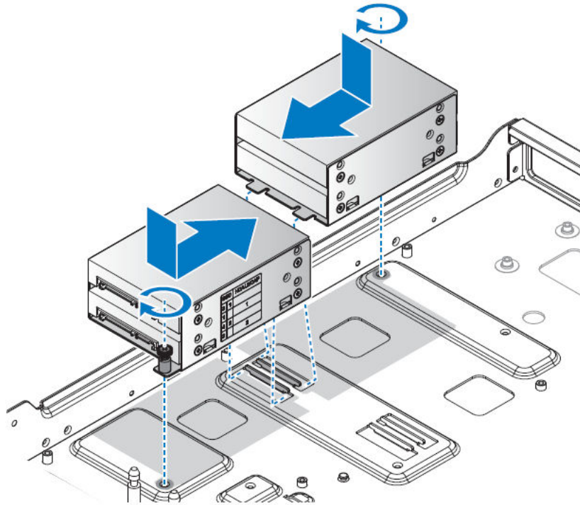
그림 24 . 2.5인치 HDD 조립품 설치
