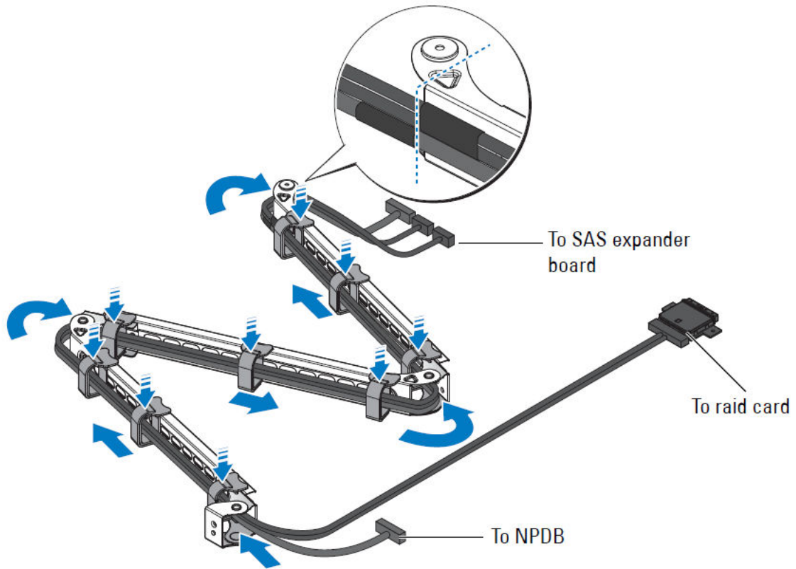
그림 150. 완료된 CMA 조립품
