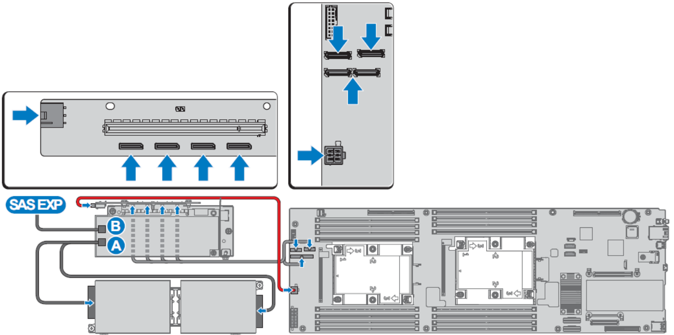
그림 138. 케이블 연결
