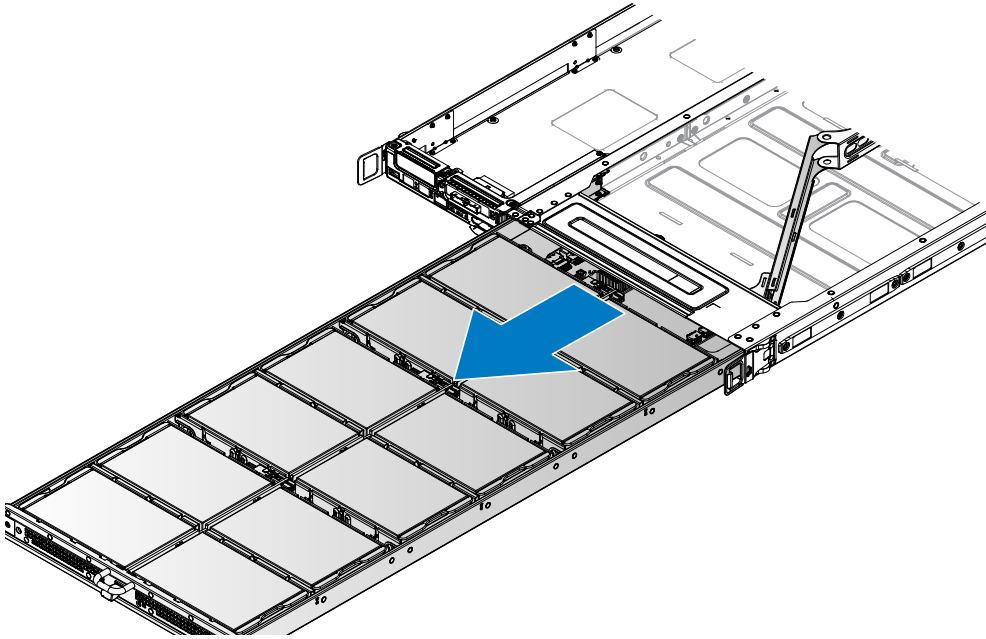
그림 26 . HDD 트레이 분리
