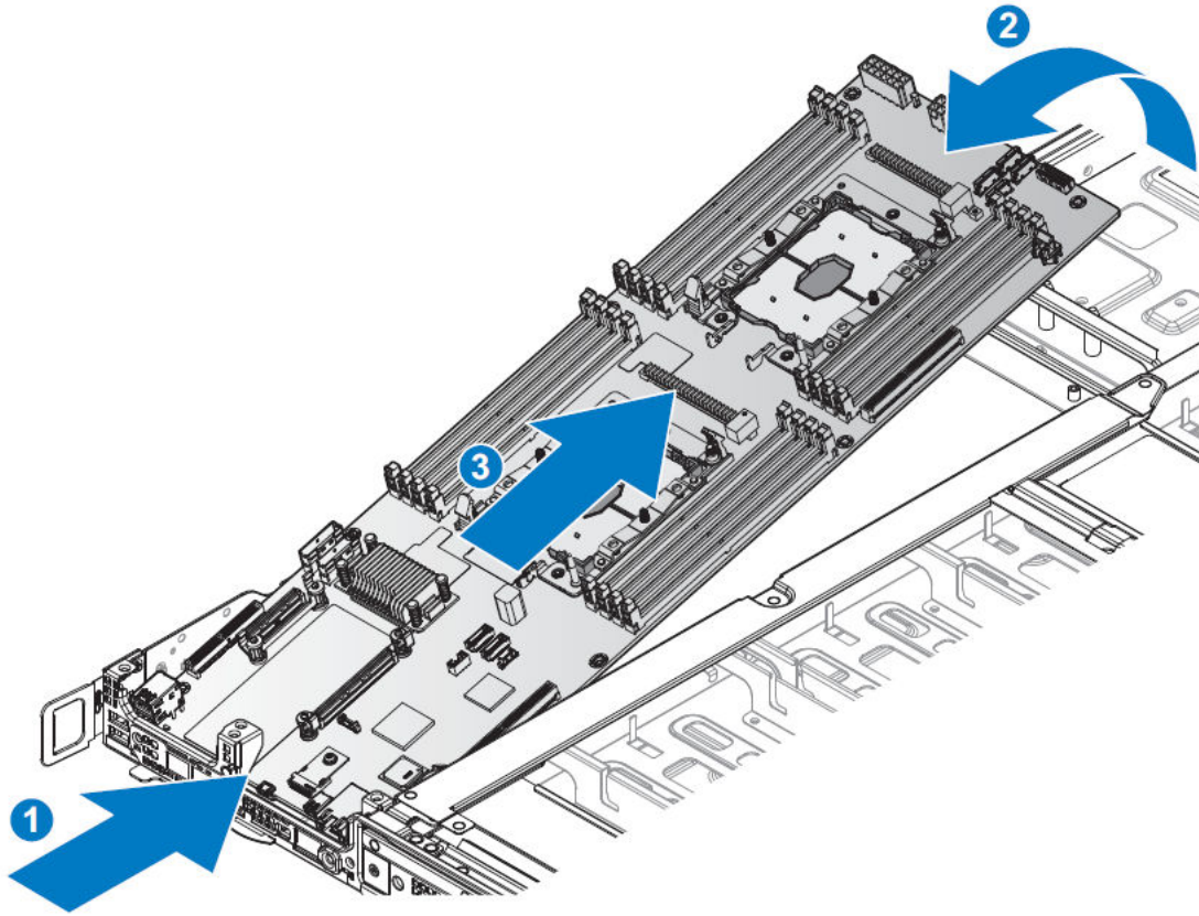
그림 43. 서버 보드 분리
