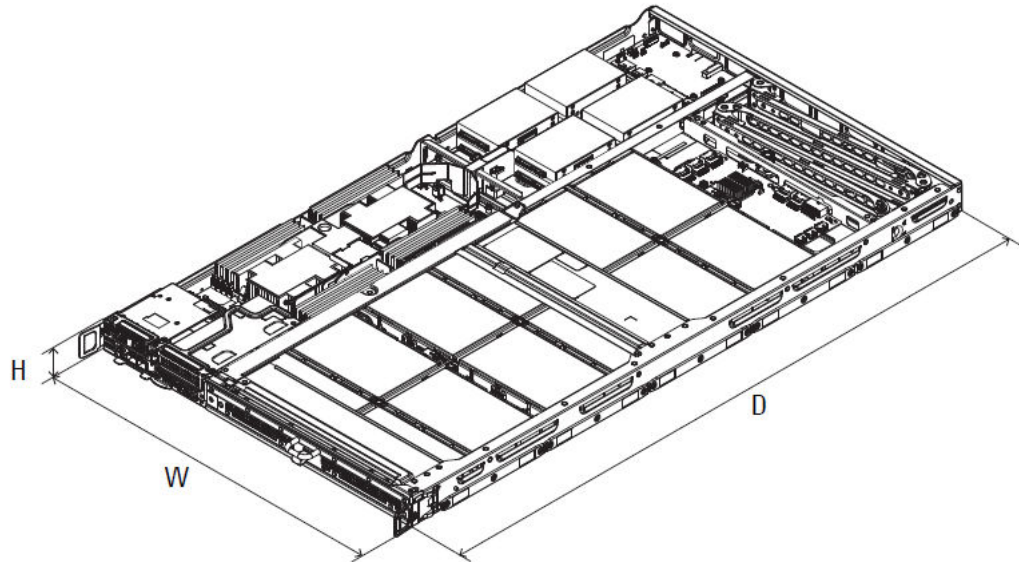
Abbildung 2. DSS 9600 – Abmessungen
