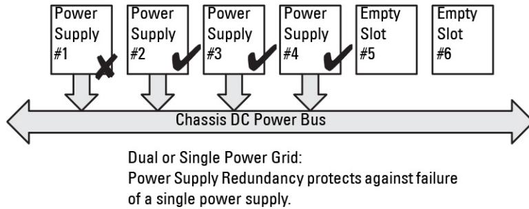
Abbildung 6. Netzteilredundanz: Insgesamt 4 Netzteileneinheiten bei Ausfall einer Netzteileneinheit.
