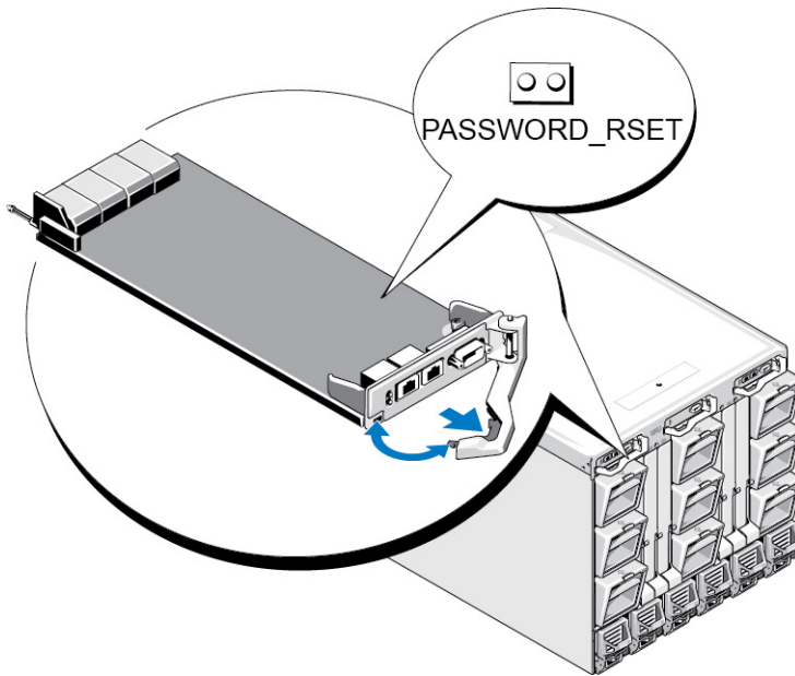
Abbildung 9. Kennwort-Reset-Jumperposition
