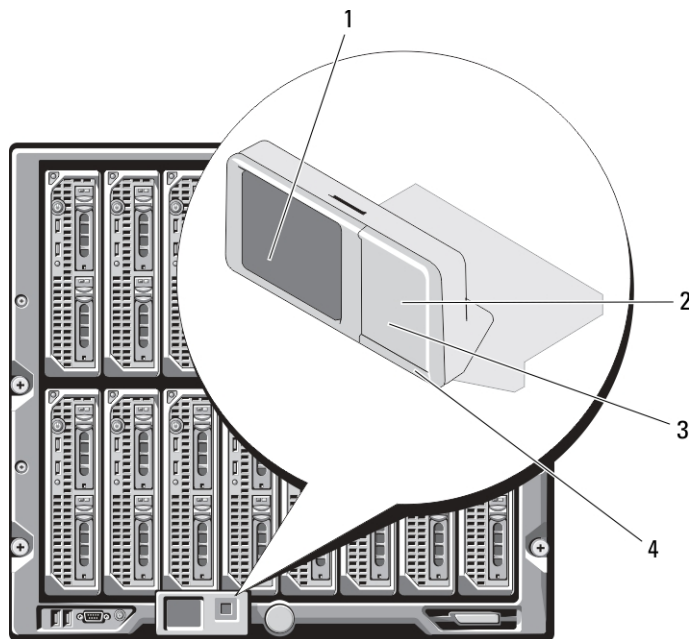
Abbildung 10. LCD-Anzeige
