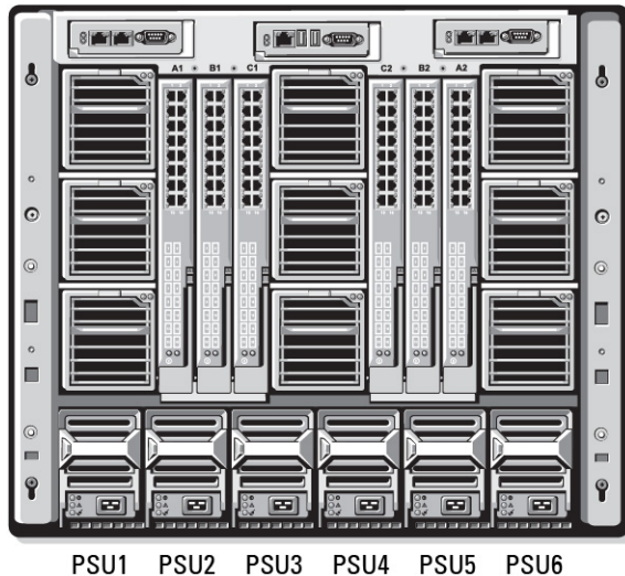
Abbildung 8. Gehäuse mit einer Konfiguration für sechs Netzteileinheiten
