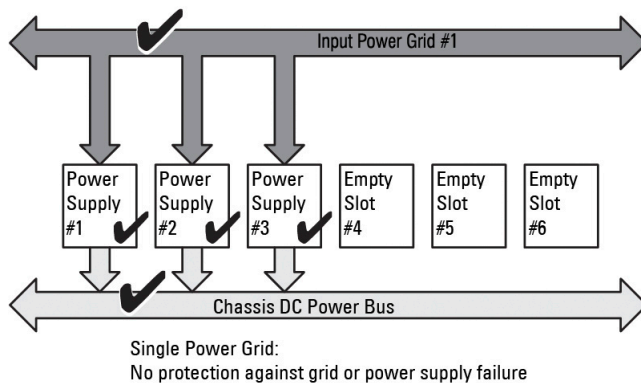
Abbildung 7. „Keine Redundanz“ bei drei Netzteileneinheiten im Gehäuse
