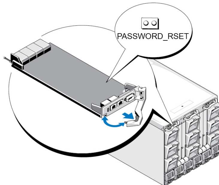
図 18. パスワードリセットジャンパーの位置
