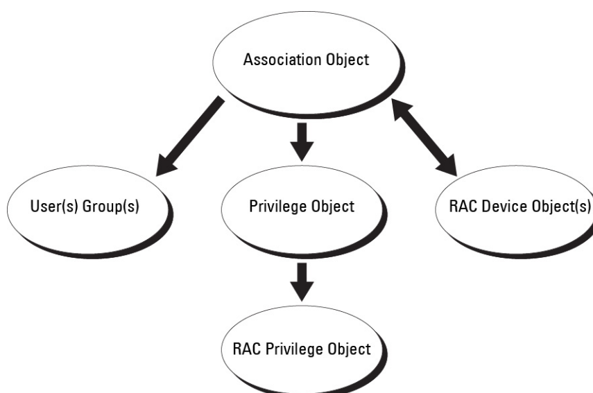
Ilustración 8. Configuración típica de los objetos de Active Directory
