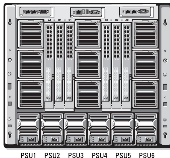
Abbildung 17. Gehäuse mit einer Konfiguration für sechs Netzteilereinheiten
