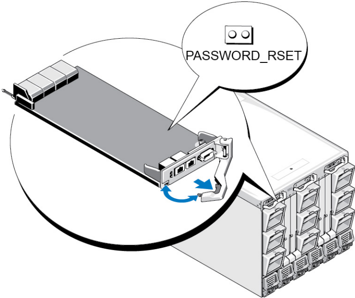
Abbildung 18. Kennwort-Reset-Jumperposition
