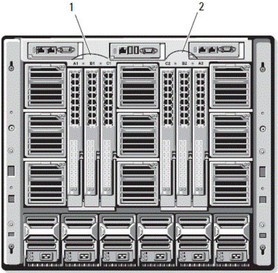
Abbildung 13. Rückansicht eines Gehäuses mit ausgewiesenen EAM-Standorten
