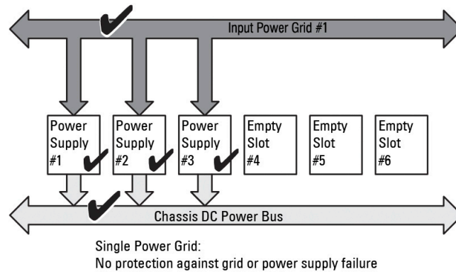
Abbildung 16. „Keine Redundanz“ bei drei Netzteileneinheiten im Gehäuse
