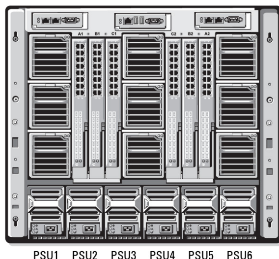
Figura 17. Configuración de chasis con seis unidades de suministro de energía
