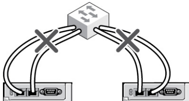
Figura 3. Cableado incorrecto para la red de la CMC: 2 CMC
