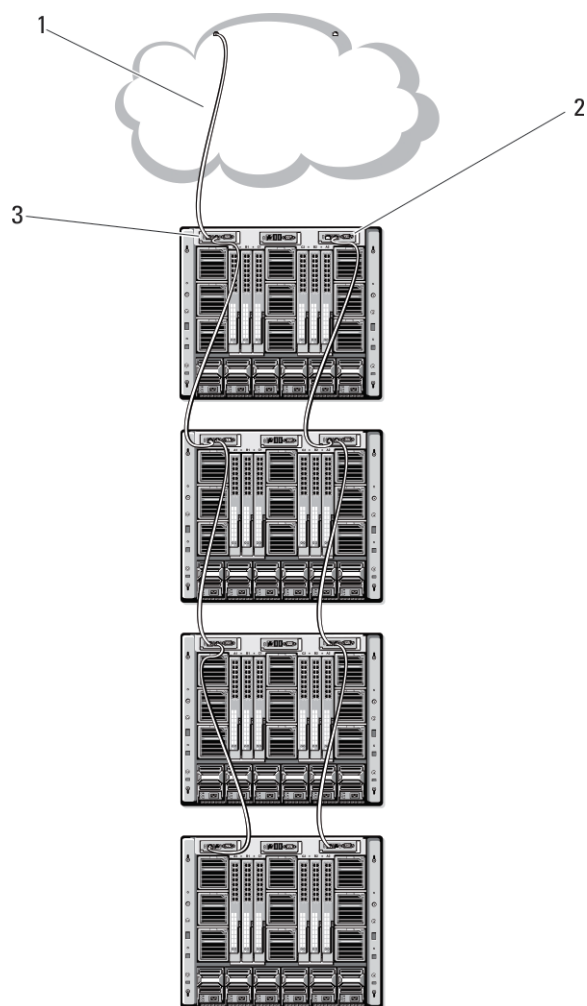
Figura 2. Conexión en cadena tipo margarita de la CMC a la red
