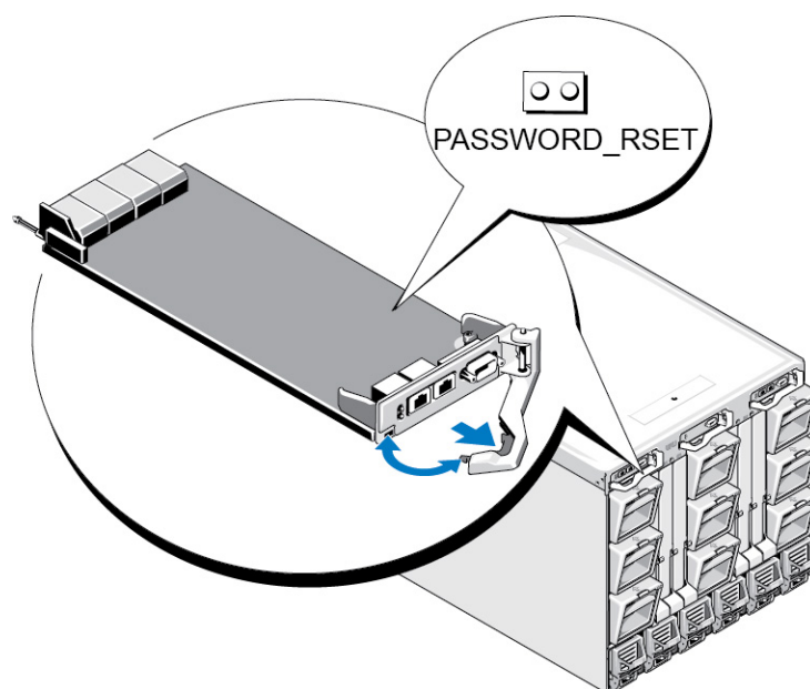
Figura 18. Ubicación del puente de restablecimiento de contraseña
