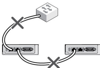
Figura 5. Cableado incorrecto para la red de la CMC: 2 CMC
