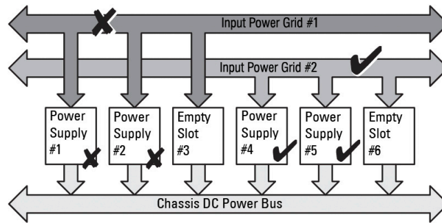
Abbildung 14. Netzteilredundanz pro Netz und ein Stromausfall in Netz 1
