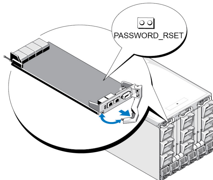
Abbildung 18. Kennwort-Reset-Jumperposition
