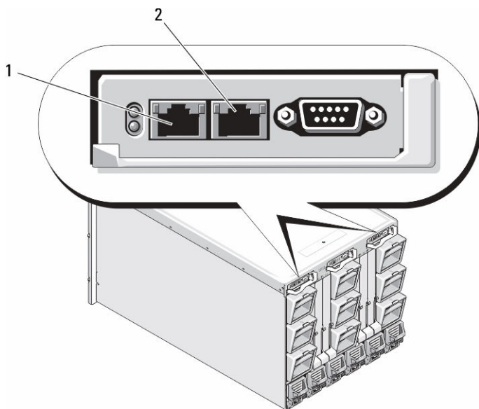
图 1: 机箱中的 CMC 插槽位置
