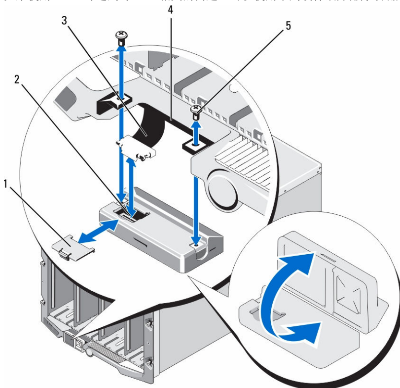
图 20: 卸下和安装 LCD 模块
