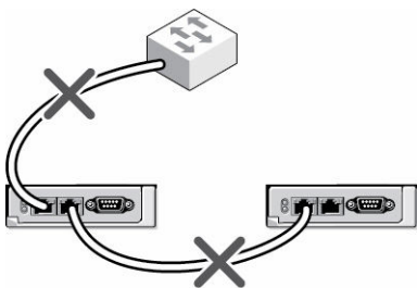
图 5: CMC 网络布线错误 - 2 个 CMC
