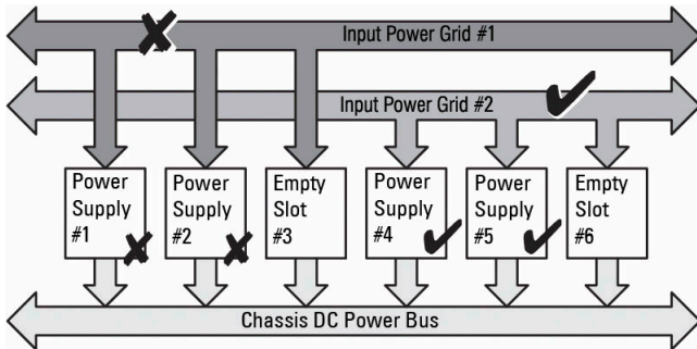
图 14: 每个电网 2 个 PSU 和电网 1 上的供电故障
