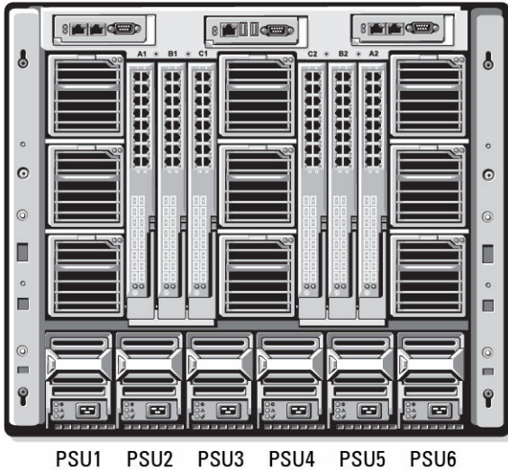
图 17: 配备六个 PSU 的机箱
