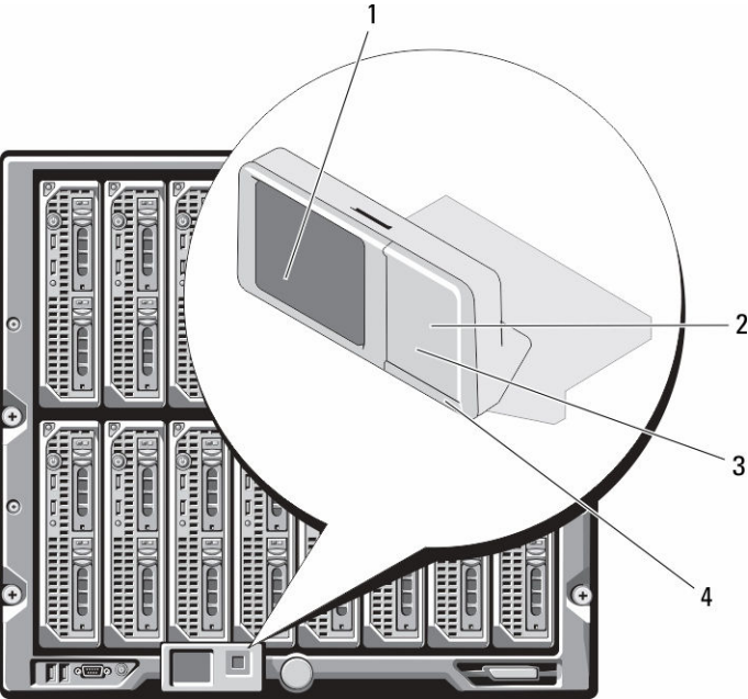
图 19: LCD 显示屏
