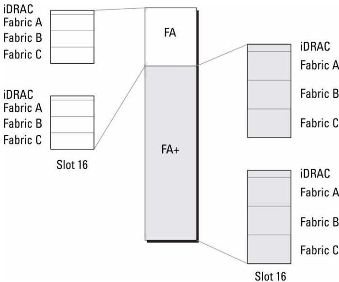
图 12: FlexAddress (FA) 和 FlexAddress Plus (FA+) 功能对比
