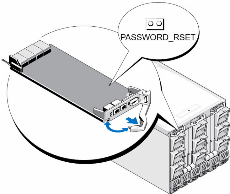
图 18: 密码重设跳线位置
