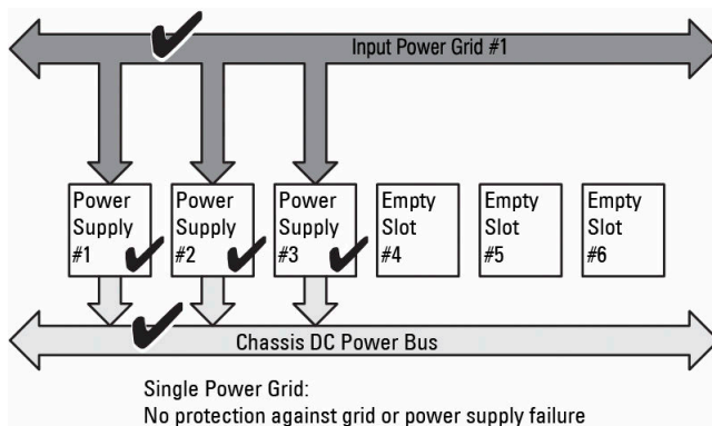
图 16: 机箱中 3 个 PSU 且无冗余
