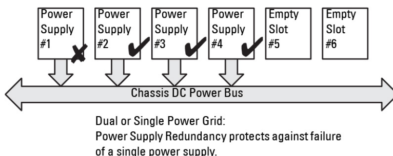
Figura 15. Redundancia de suministro de energía: total de 4 unidades de suministro de energía con la falla de una unidad
