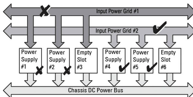
Figura 14. Unidades de suministro de energía por cada red eléctrica y una falla de alimentación en la red eléctrica 1
