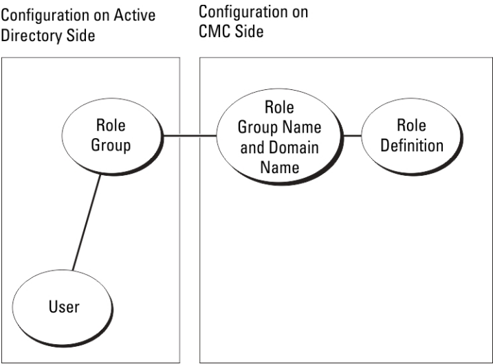
Figura 7. Configuración de la CMC con el esquema estándar de Active Directory
