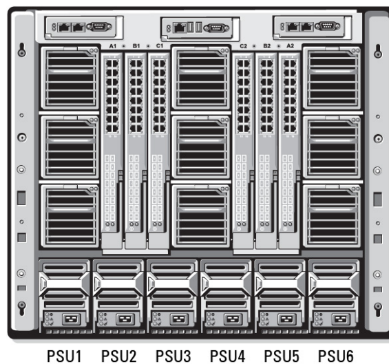
Figura 17. Configuración de chasis con seis unidades de suministro de energía
