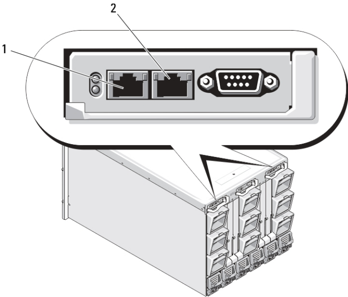
Figura 1. Ubicación de las ranuras de la CMC en el chasis
