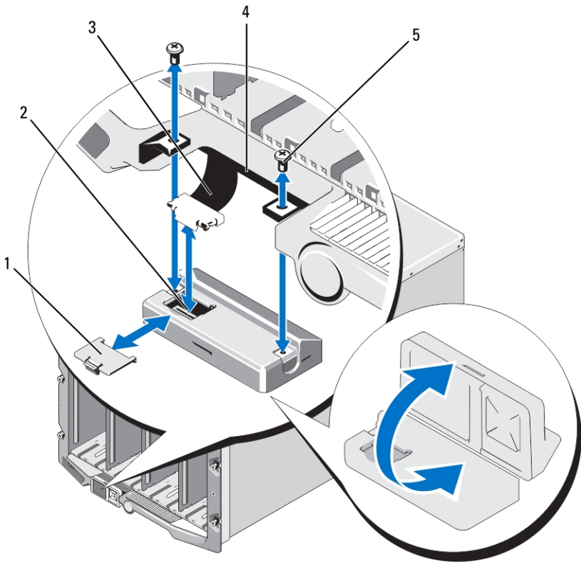
Figura 20. Extracción e instalación del módulo LCD
