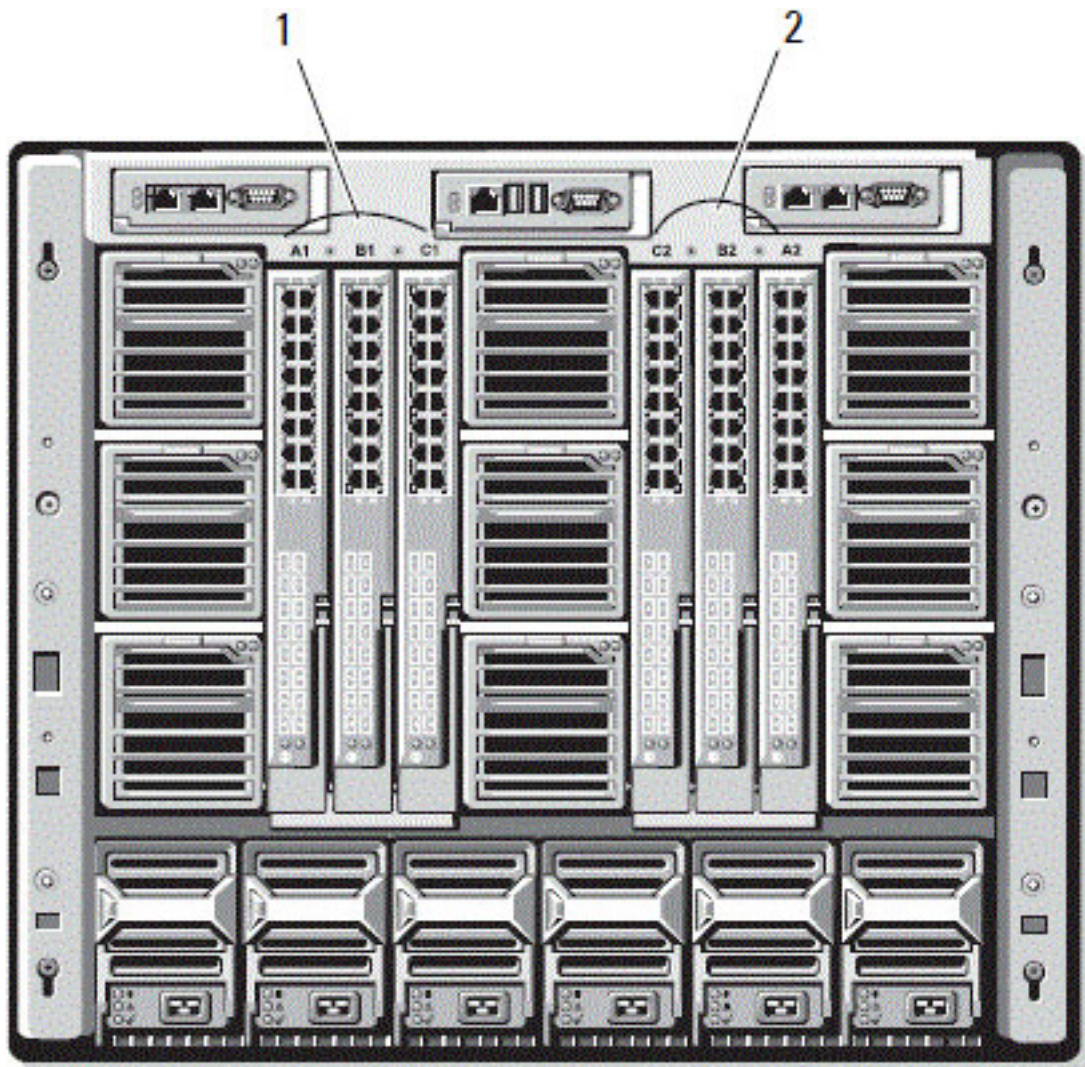
Figura 13. Vista posterior de un chasis, que muestra la ubicación de los módulos de E/S
