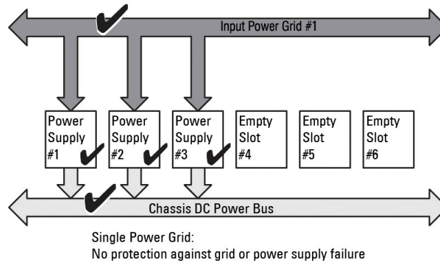
Figura 16. Sin redundancia con tres unidades de suministro de energía en el chasis
