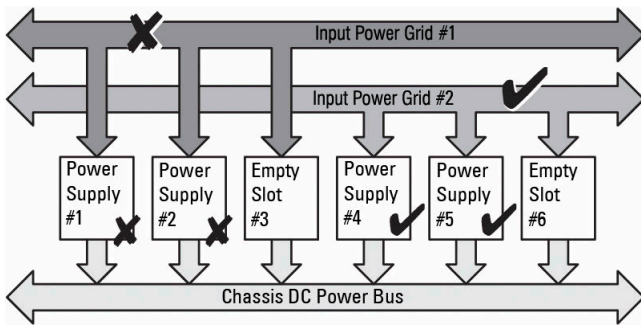
Ilustración 14. Unidades de suministro de energía por cada red eléctrica y una falla de alimentación en la red eléctrica 1
