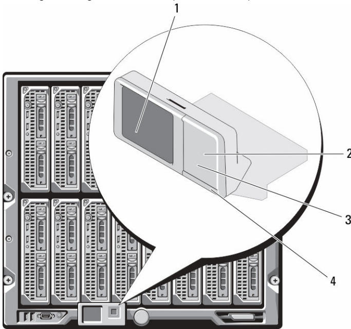
Ilustración 19. Pantalla LCD
