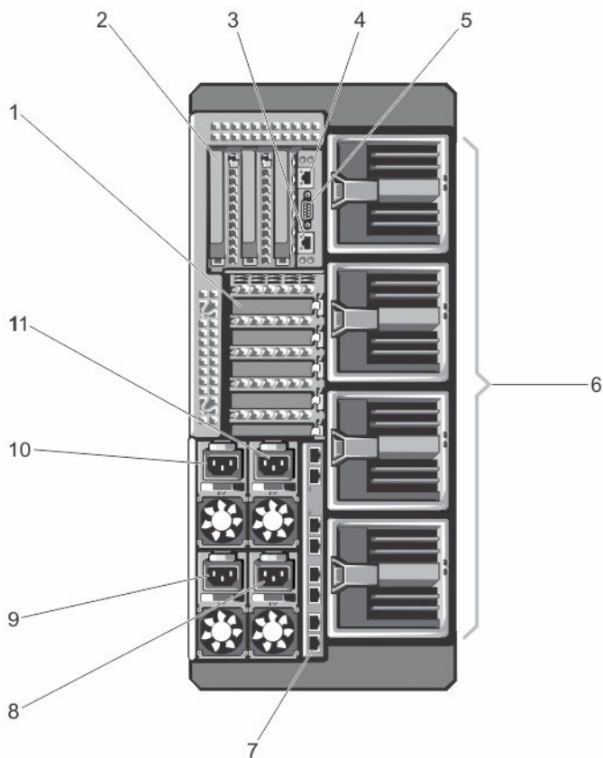
図 2. CMC の背面パネル
