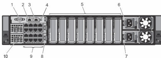
図 1. シャーシの背面パネル
