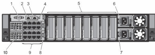
Figure 1. Panneau arrière du châssis
