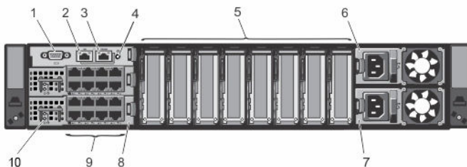
Abbildung 1. Rückseite des Gehäuses
