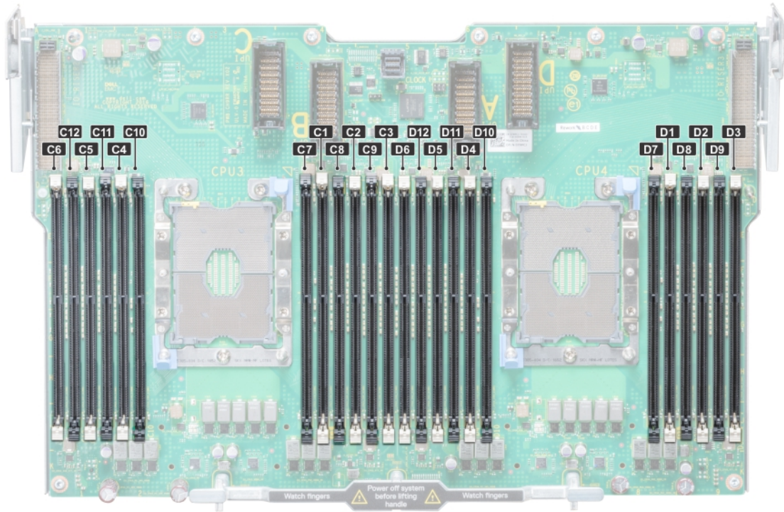
图 35: 处理器扩充模块上的内存插槽位置
