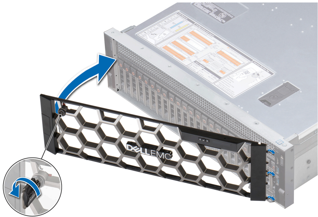
图 14: 安装可选的前挡板与 LCD 面板
