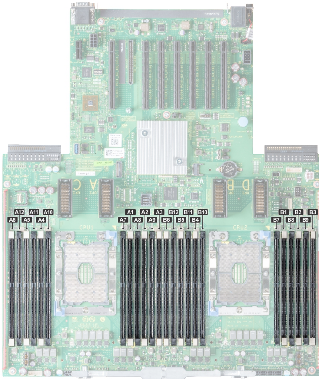
Figura 34. Ubicación de los zócalos de memoria
