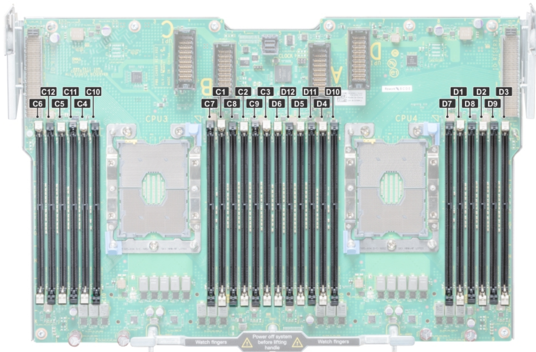
Figura 35. Ubicación de los zócalos de memoria en el módulo de expansión del procesador
