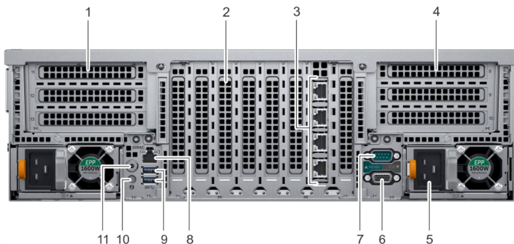
Figura 6. Características de la vista posterior
