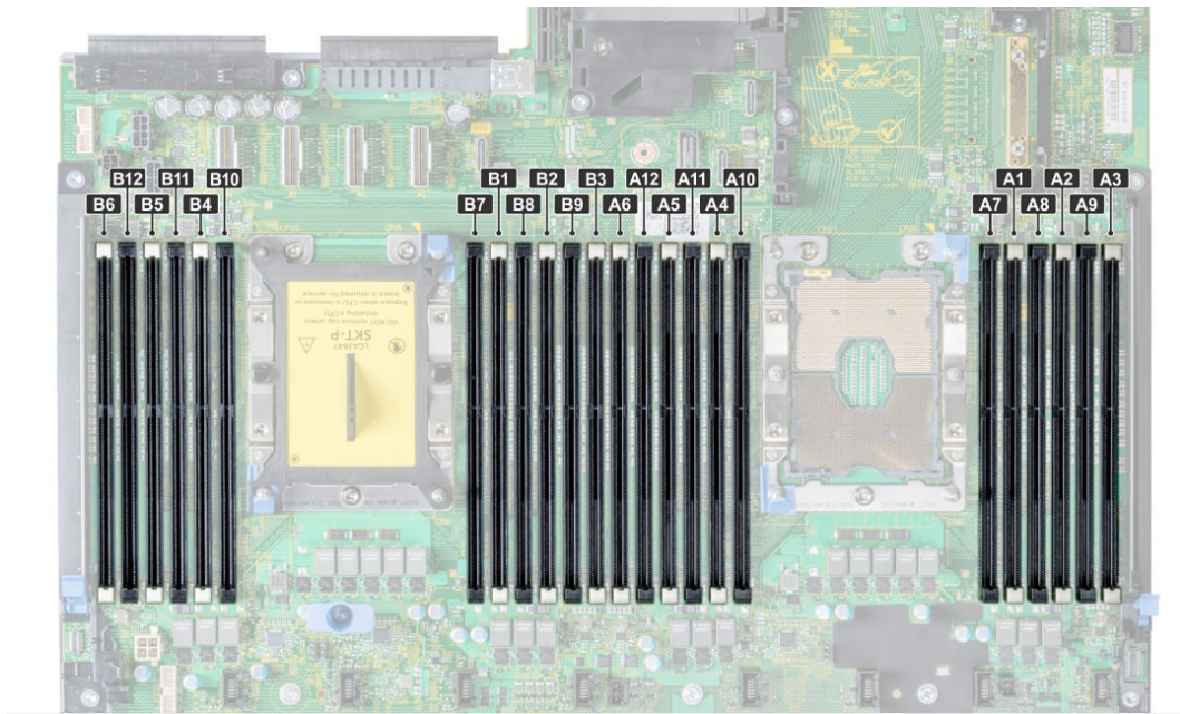
图 1: R740/R740XD 的内存布局
