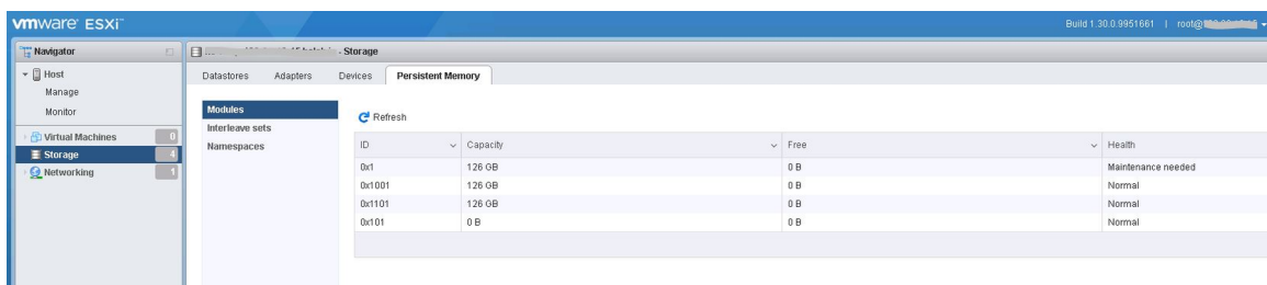
Abbildung 28. PMEM-Funktionswarnung
