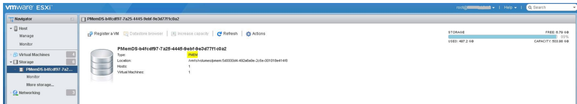
Abbildung 27. PMEM-Datenspeicher
