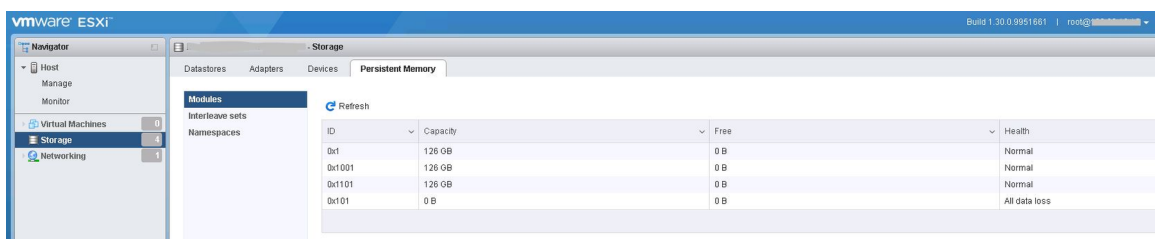
Abbildung 29. PMEM-Multibit-Fehler
