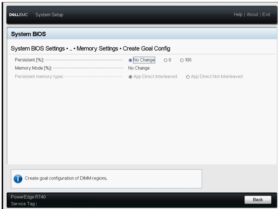
Abbildung 4. Zielkonfiguration
