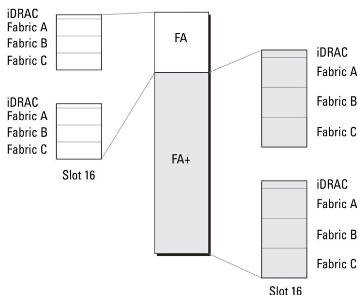
図 12. FlexAddress ( FA ) と FlexPlusAddress ( FA+ ) の機能
