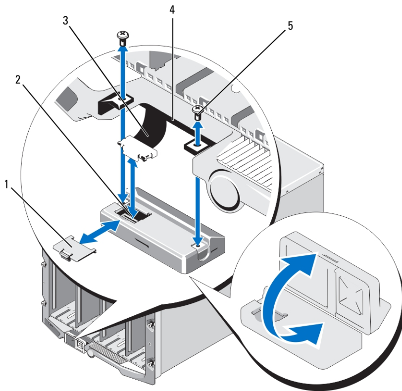
図 20. LCD モジュールの取り外しと取り付け
