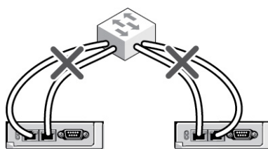
図 3. CMC ネットワークの誤ったケーブル接続 - CMC が 2 つ
