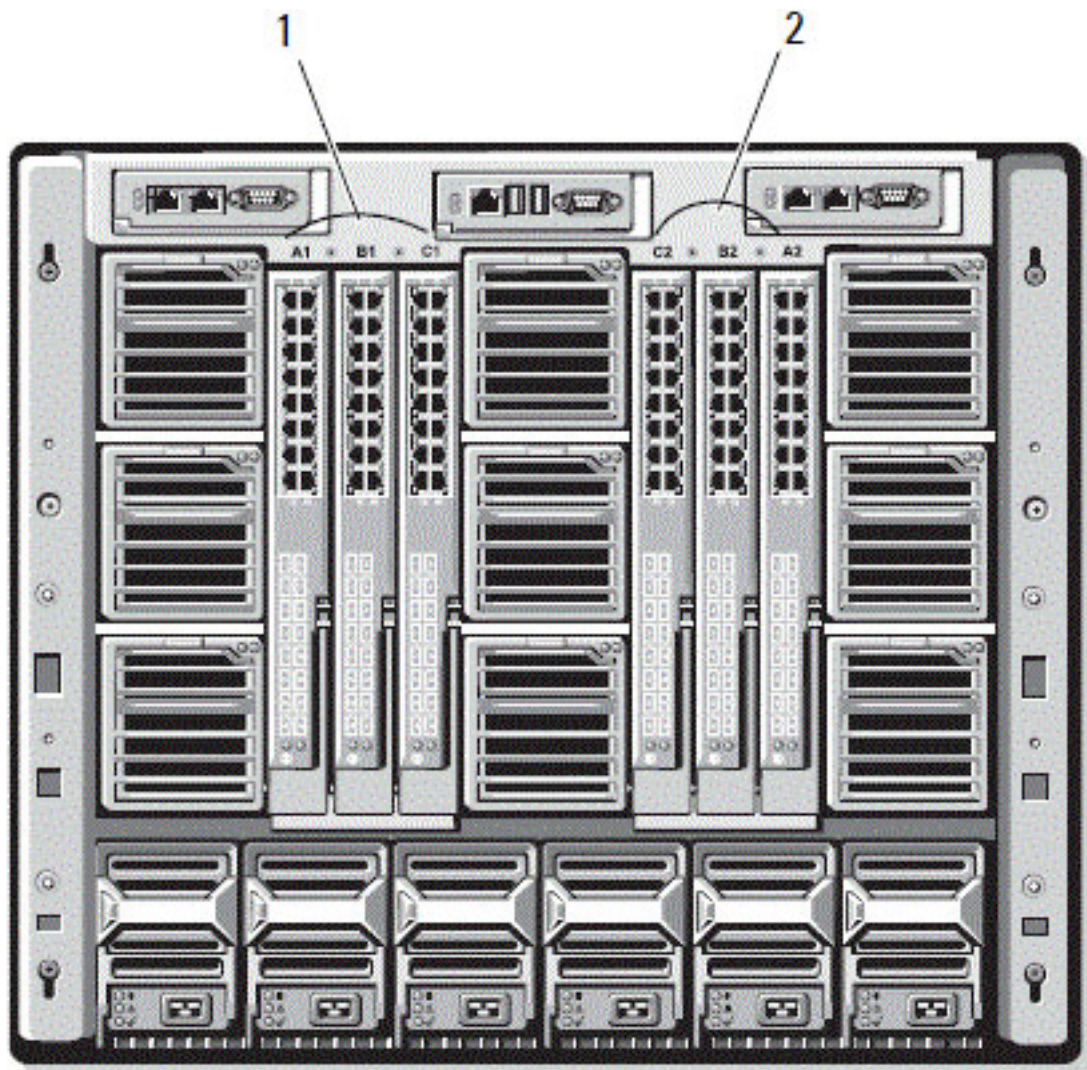
図 13. IOM の位置を示すシャーシの背面図
