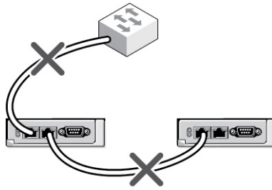
図 5. CMC ネットワークの誤ったケーブル接続 - CMC が 2 つ
