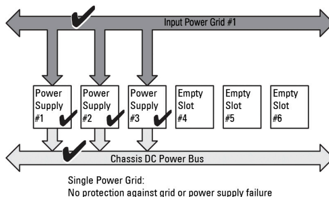
図 16. 3 台の PSU を備えたシャーシでの冗長性なし
