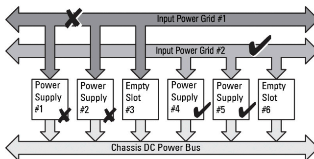
図 14. グリッドにつき PSU が 2 台、グリッド 1 で電源障害
