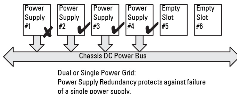
図 15. 電源装置の冗長性：合計 4 台の PSU があり、そのうち 1 台が故障。
