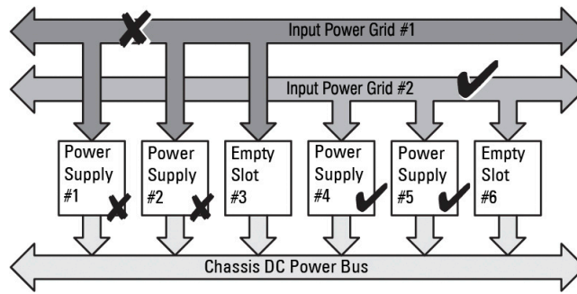
Figure 14. blocs d'alimentation par réseau électrique avec une panne électrique sur le réseau 1
