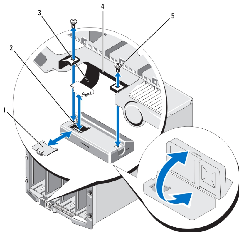
Abbildung 20. LCD-Modul entfernen und installieren
