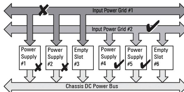
Abbildung 14. Netzteileneinheiten pro Netz und ein Stromausfall in Netz 1
