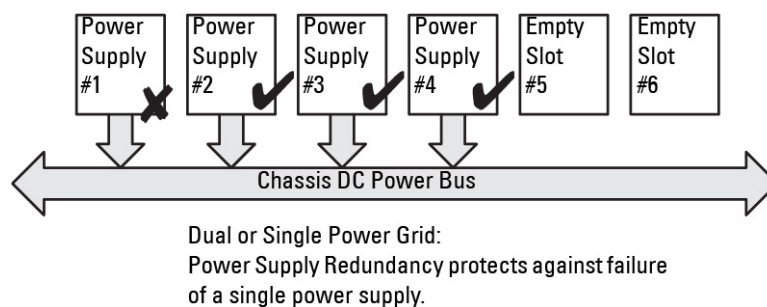
Abbildung 15. Netzteilredundanz: Insgesamt 4 Netzteilereinheiten bei Ausfall einer Netzteilereinheit.
