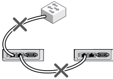
Abbildung 5. Inkorrekte Verkabelung für CMC-Netzwerk - 2 CMCs
