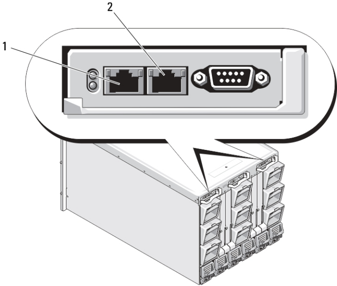
Abbildung 1. Positionen der CMC-Steckplätze im Gehäuse
