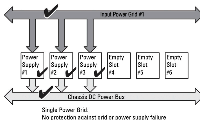
Abbildung 16. „Keine Redundanz“ bei drei Netzteilereinheiten im Gehäuse
