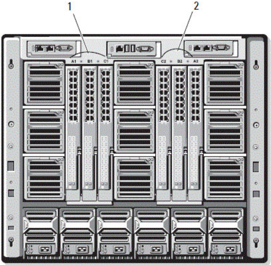
Abbildung 13. Rückansicht eines Gehäuses mit ausgewiesenen EAM-Standorten
