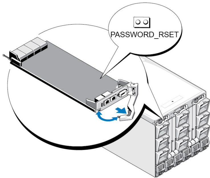
Abbildung 18. Kennwort-Reset-Jumperposition
