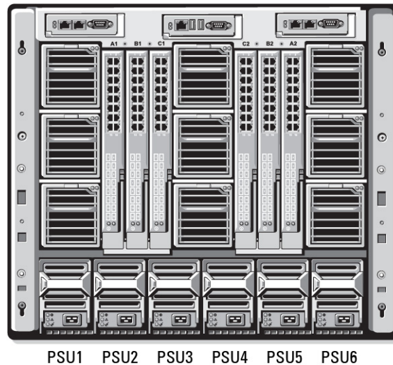
Abbildung 17. Gehäuse mit einer Konfiguration für sechs Netzteileneinheiten
