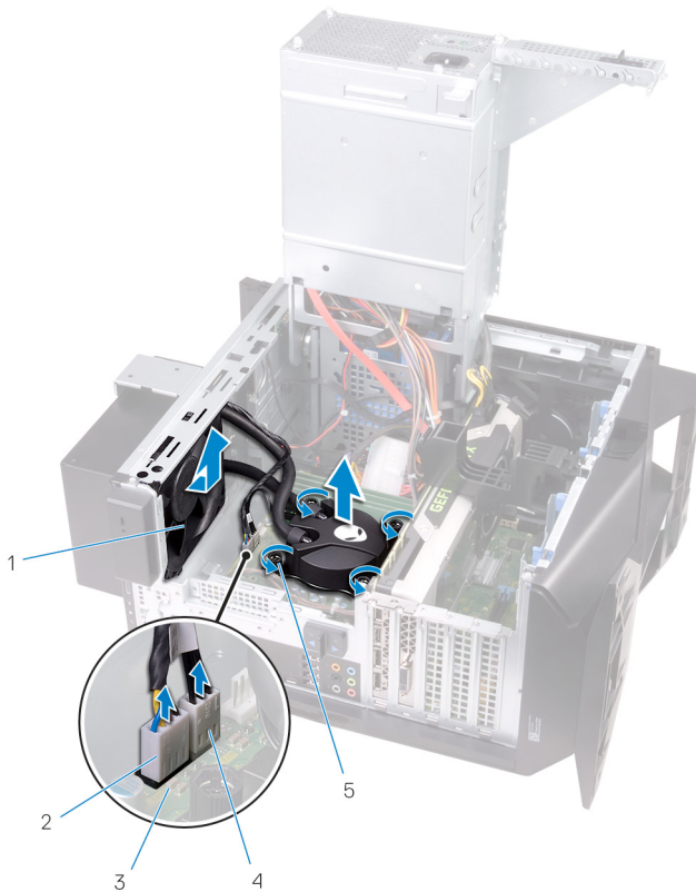
21. ábra. A processzorhűtő egység eltávolítása
