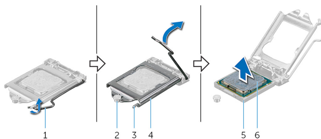
31. ábra. A processzor eltávolítása
