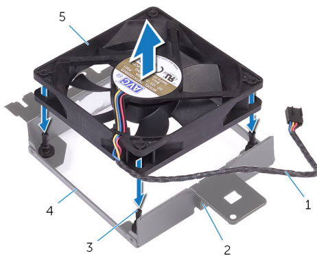
40. ábra. A felső házventilátor eltávolítása
