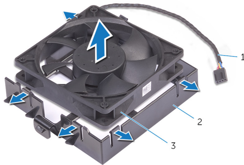
38. ábra. A házventilátor eltávolítása
