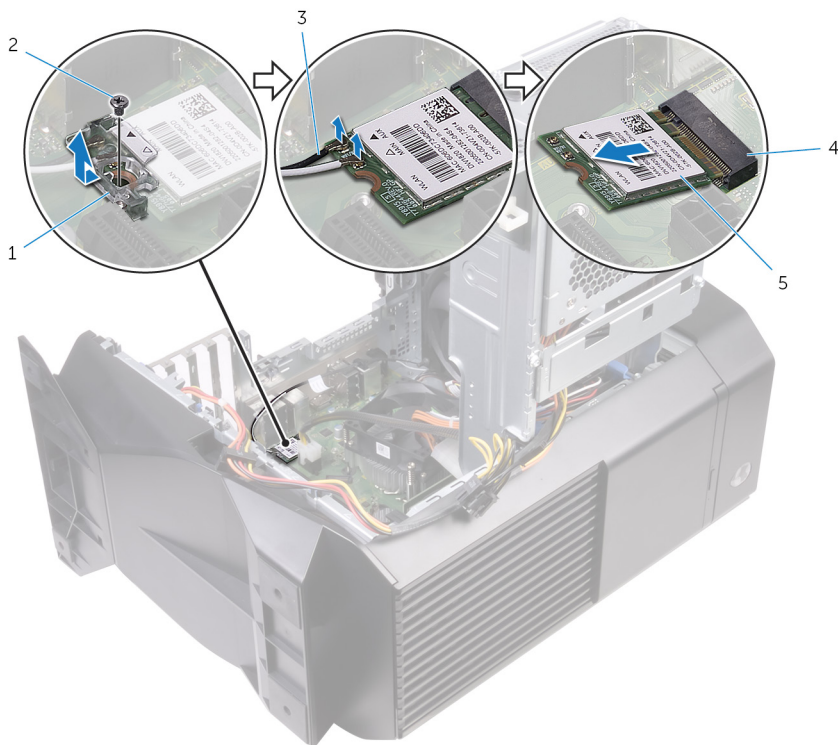
33. ábra. A vezeték nélküli kártya eltávolítása
