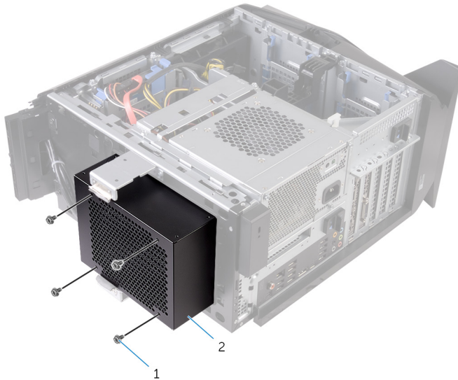
19. ábra. A processzorhűtő egység eltávolítása
