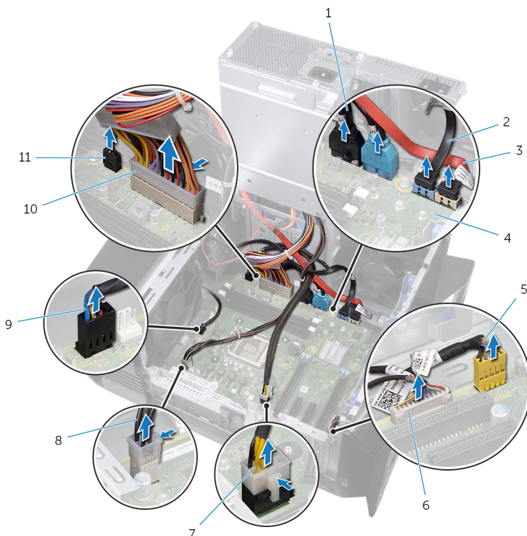
50. ábra. Az alaplapi eltávolítása
