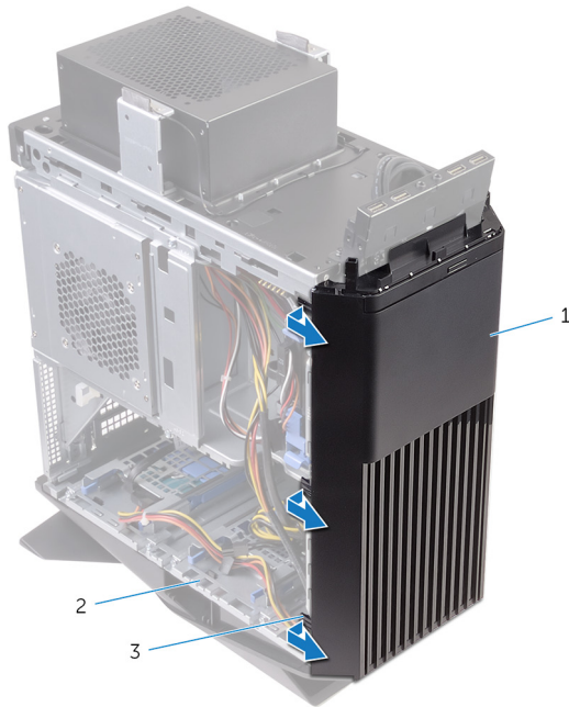
45. ábra. Az előlső előlap eltávolítása
