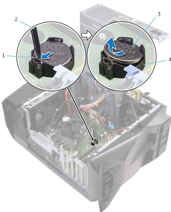
24. ábra. A gombelem eltávolítása
