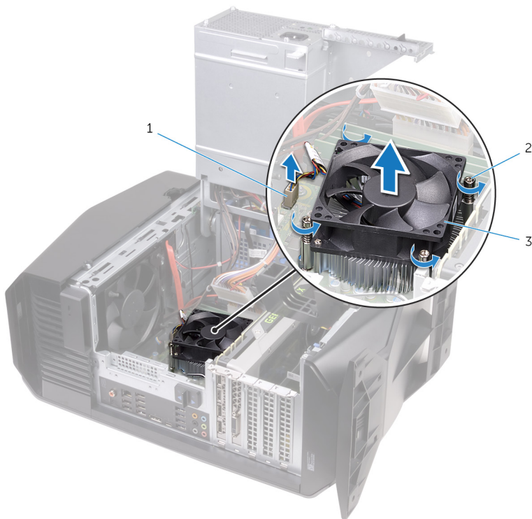
30. ábra. A processzorventilátor és a hűtőborda egység eltávolítása
