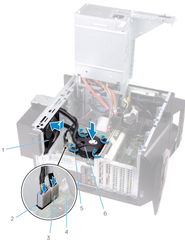
22. ábra. A processzorhűtő egység visszahelyezése
