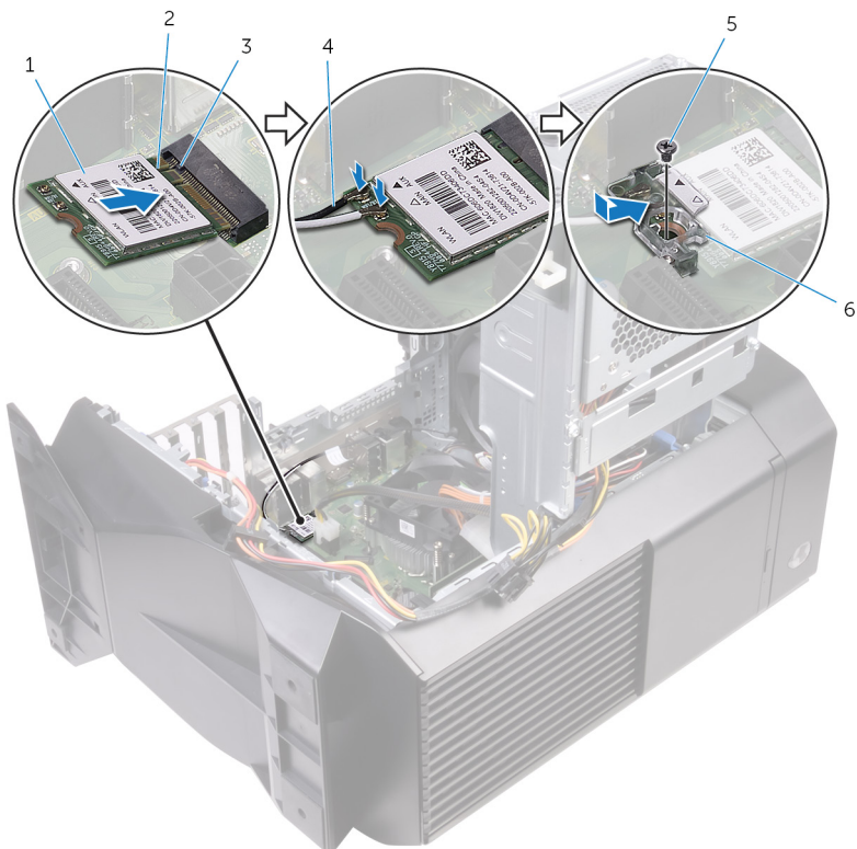
34. ábra. A vezeték nélküli kártya visszahelyezése
