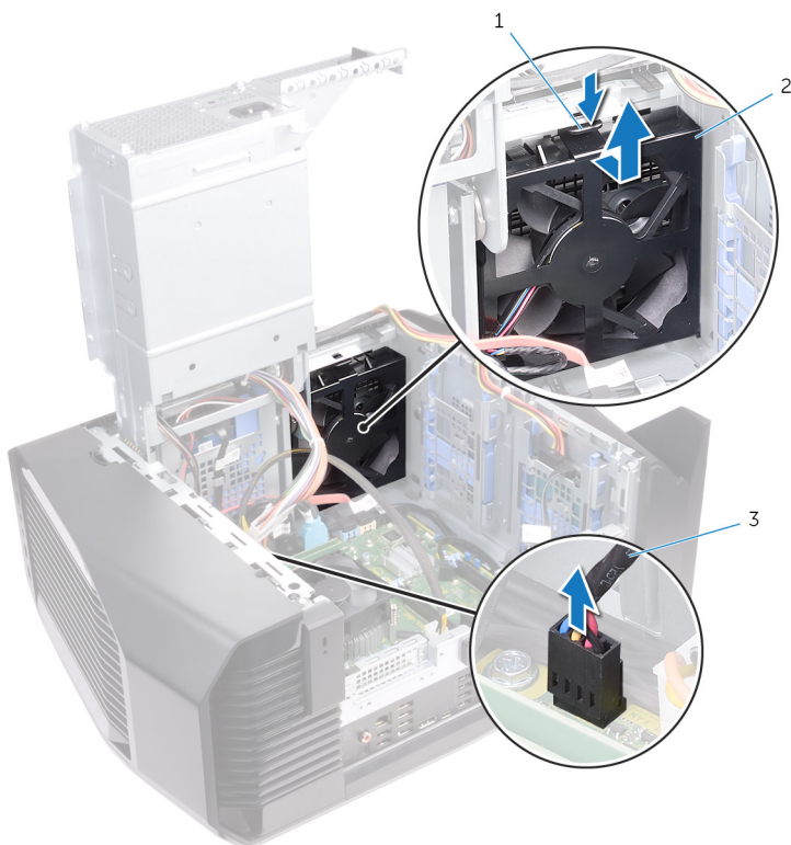
37. ábra. A házventilátor eltávolítása
