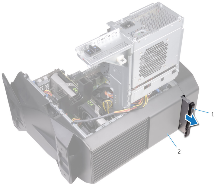
42. ábra. Az optikai meghajtó eltávolítása
