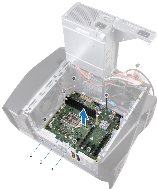
51. ábra. Az alaplapi eltávolítása
