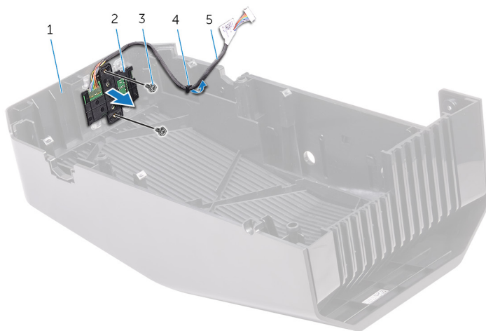
47. ábra. A bekapcsológomb modul eltávolítása
