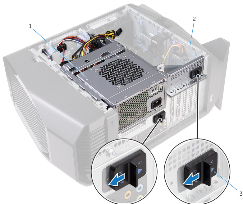
18. ábra. A tápegységtartó keret kioldóreteszeinek elcsúsztatása
