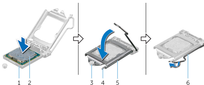
32. ábra. A processzor visszahelyezése
