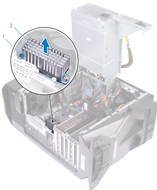
20. ábra. A VR-hűtőborda eltávolítása
