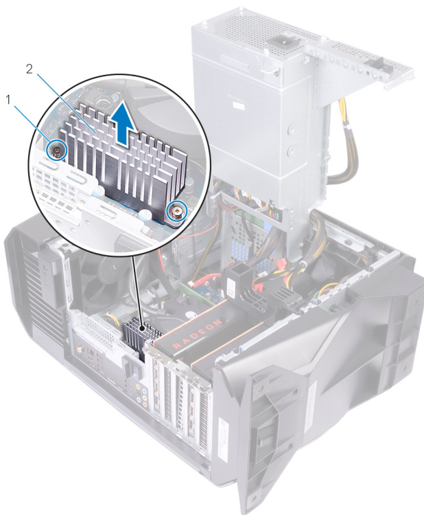
29. ábra. A VR-hűtőborda eltávolítása
