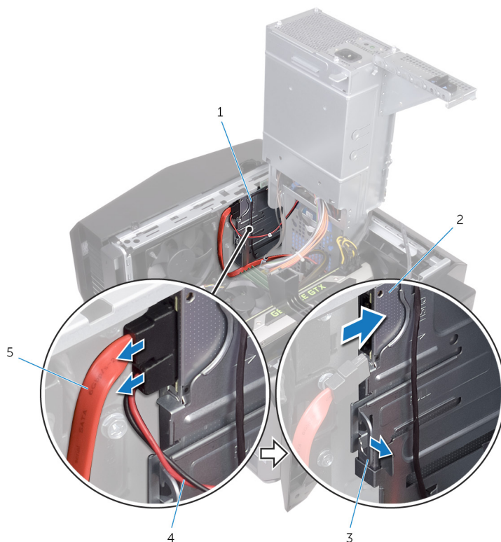
41. ábra. A táp- és az adatkábel leválasztása
