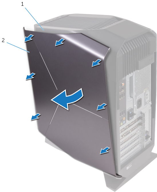
4. ábra. A jobb oldali burkolat eltávolítása
