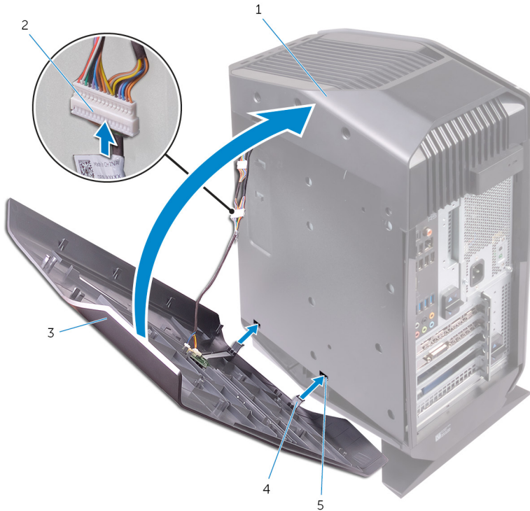
6. ábra. A világítás kábelének csatlakoztatása
