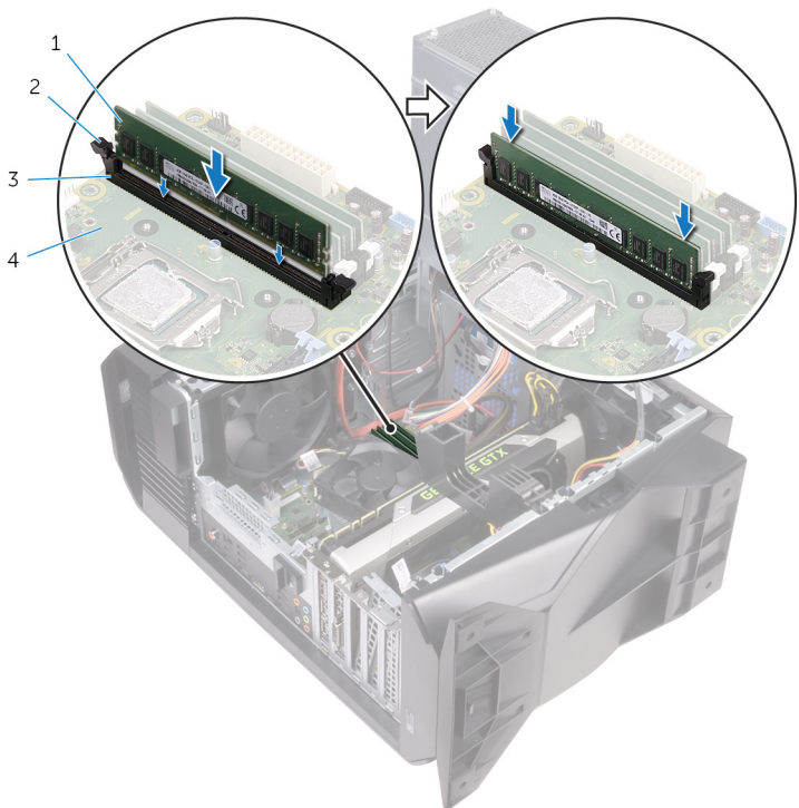
26. ábra. A memóriamodul visszahelyezése
