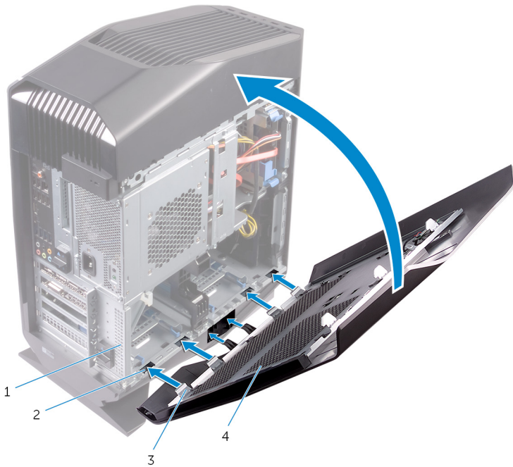
3. ábra. A bal oldali burkolat visszahelyezése
