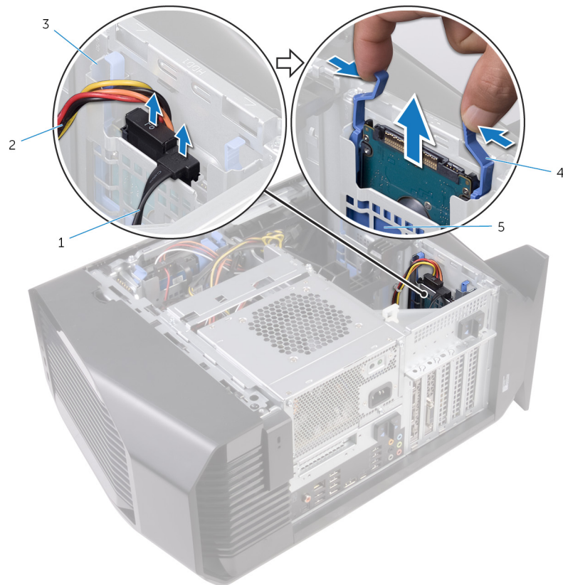
Abbildung 15. Entfernen des Festplattenlaufwerks
