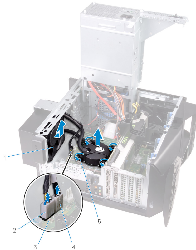
Abbildung 26. Entfernen der Prozessorkühlung-Baugruppe
