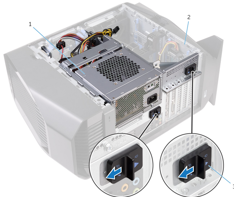
Abbildung 23. Schieben der Freigaberiegel des Netzteilgehäuses
