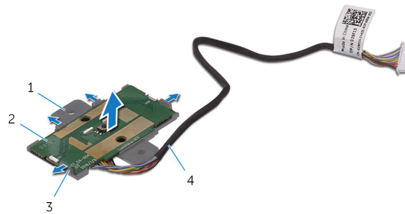
Abbildung 53. Entfernen des Betriebsschaltermoduls
