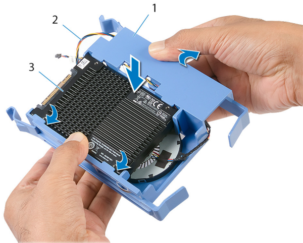
Abbildung 19. Einsetzen des U.2-SSD-Laufwerks
