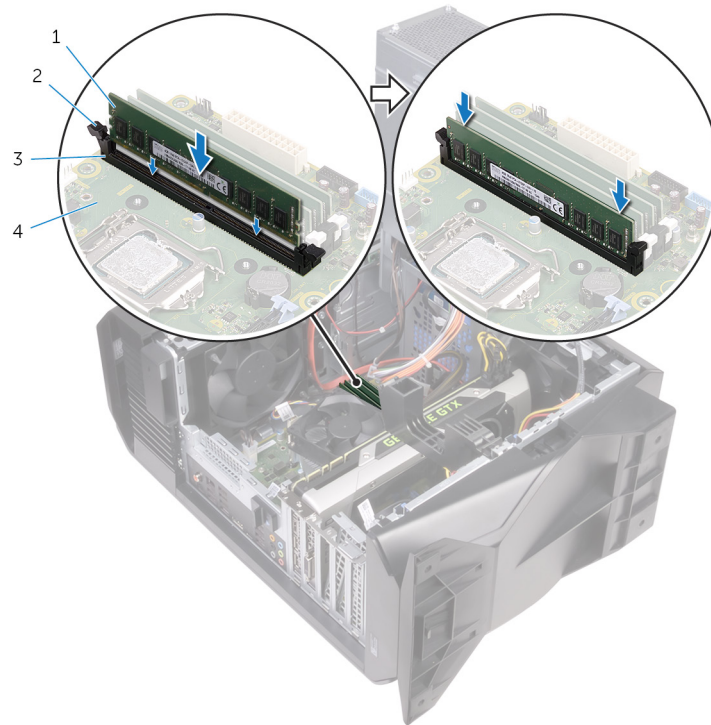
Abbildung 31. Austauschen des Speichermoduls
