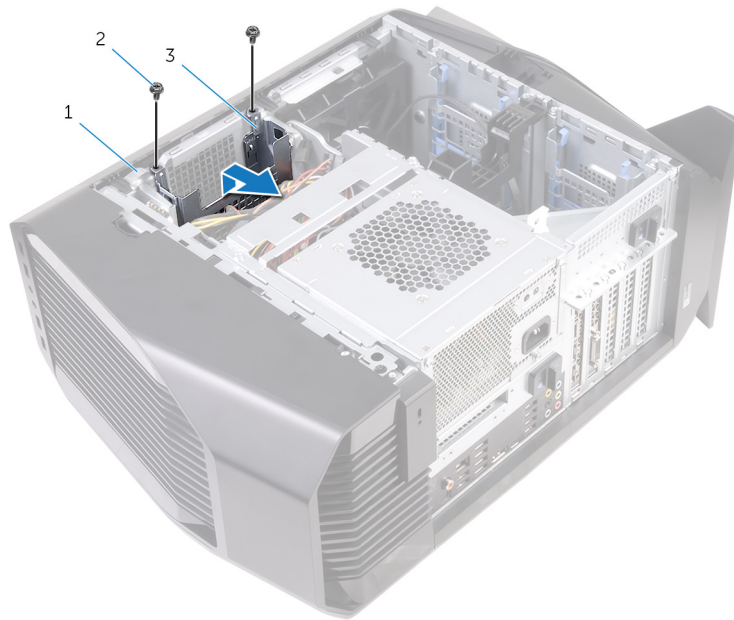
Abbildung 22. Entfernen des Laufwerksgehäuses
