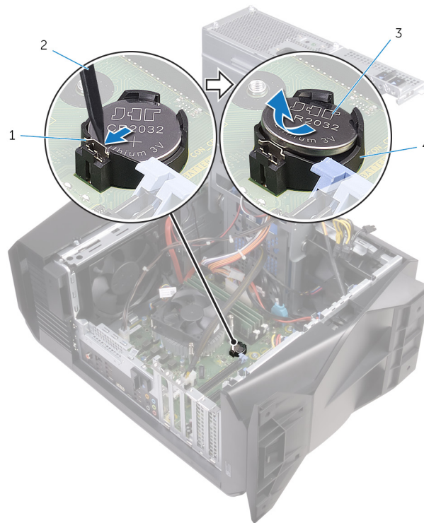
Abbildung 29. Entfernen der Knopfzellenbatterie
