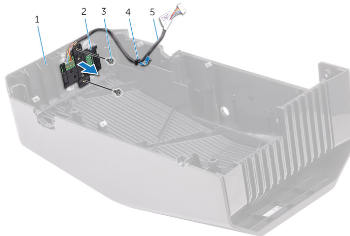
Abbildung 52. Entfernen des Betriebsschaltermoduls
