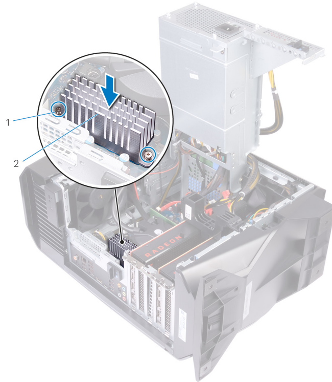
Abbildung 28. Wiedereinbauen des VR-Kühlkörpers
