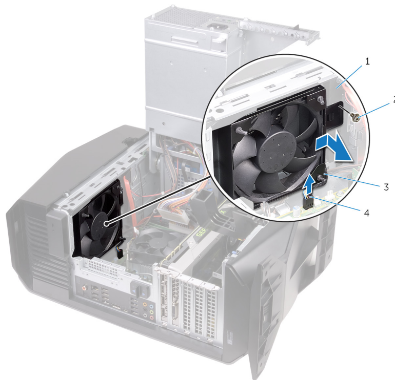
Abbildung 44. Entfernen des oberen Gehäuselüfters
