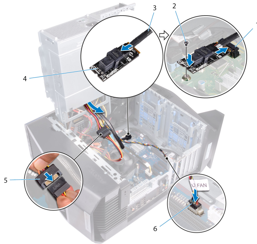
Abbildung 20. Anschließen der Kabel
