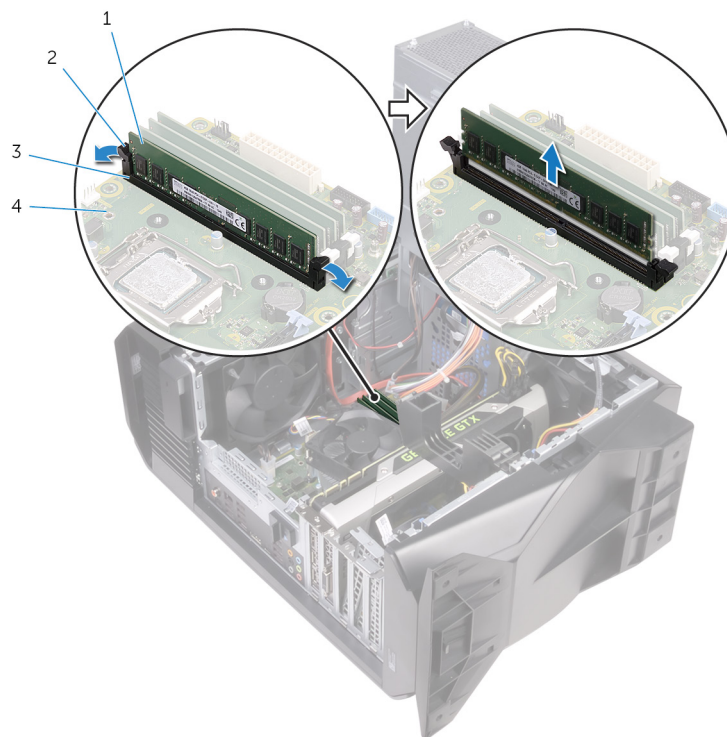
Abbildung 30. Entfernen des Speichermoduls
