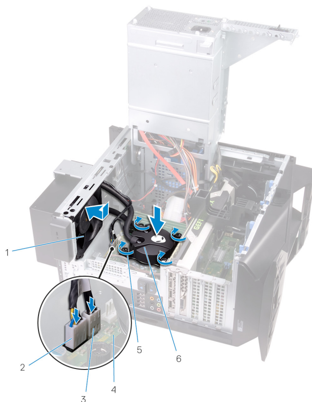
Abbildung 27. Ersetzen der Prozessorkühlung-Baugruppe
