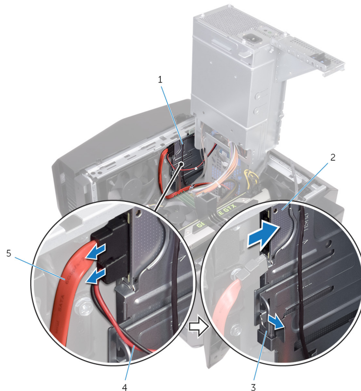
Abbildung 46. Entfernen der Strom- und Datenkabels
