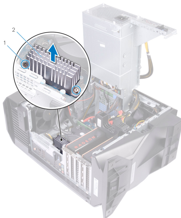
Abbildung 25. Entfernen des VR-Kühlkörpers
