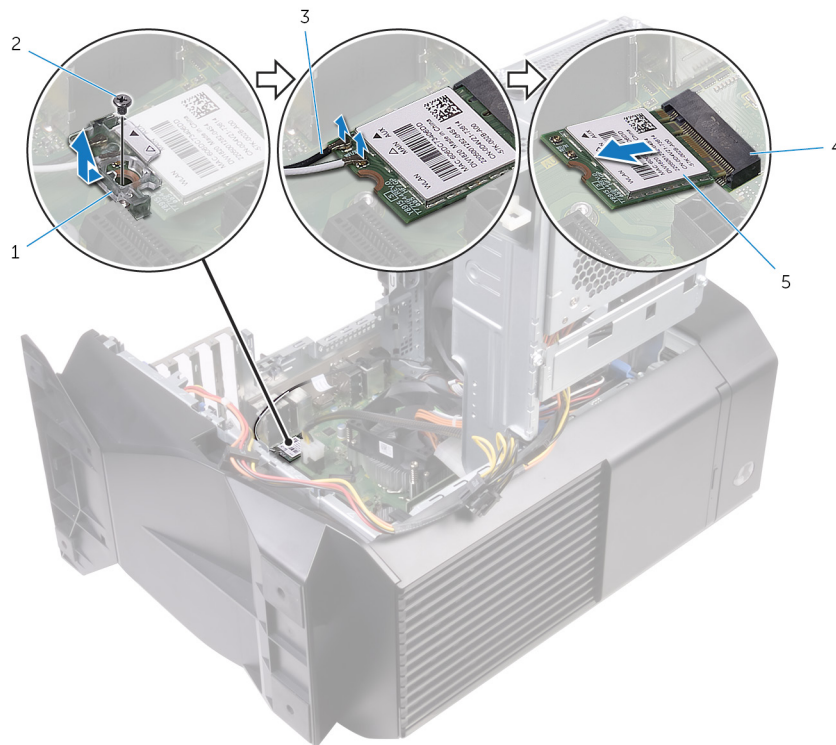
Abbildung 38. Entfernen der Wireless-Karte
