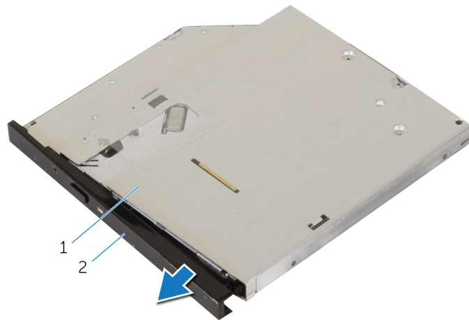
Abbildung 49. Entfernen des optischen Laufwerks
