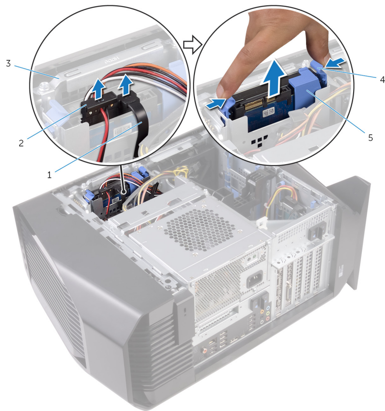
Abbildung 17. Entfernen des Festplattenlaufwerks
