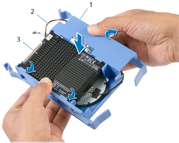
Abbildung 18. Einsetzen des U.2-SSD-Laufwerks
