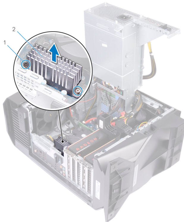
Abbildung 34. Entfernen des VR-Kühlkörpers
