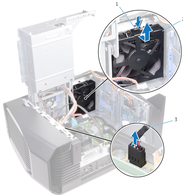
Abbildung 42. Entfernen des Gehäuselüfters
