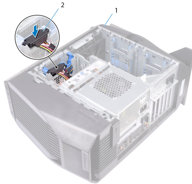
Abbildung 21. Anschließen des Stromkabels
