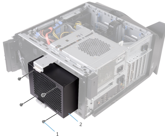
Abbildung 24. Entfernen der Prozessorkühlung-Baugruppe
