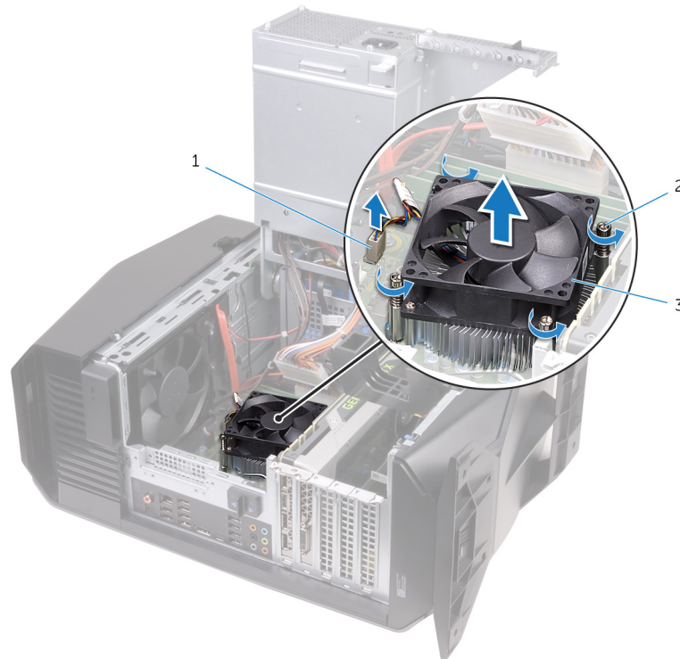
Abbildung 35. Entfernen der Prozessorlüfter- und Kühlkörperbaugruppe
