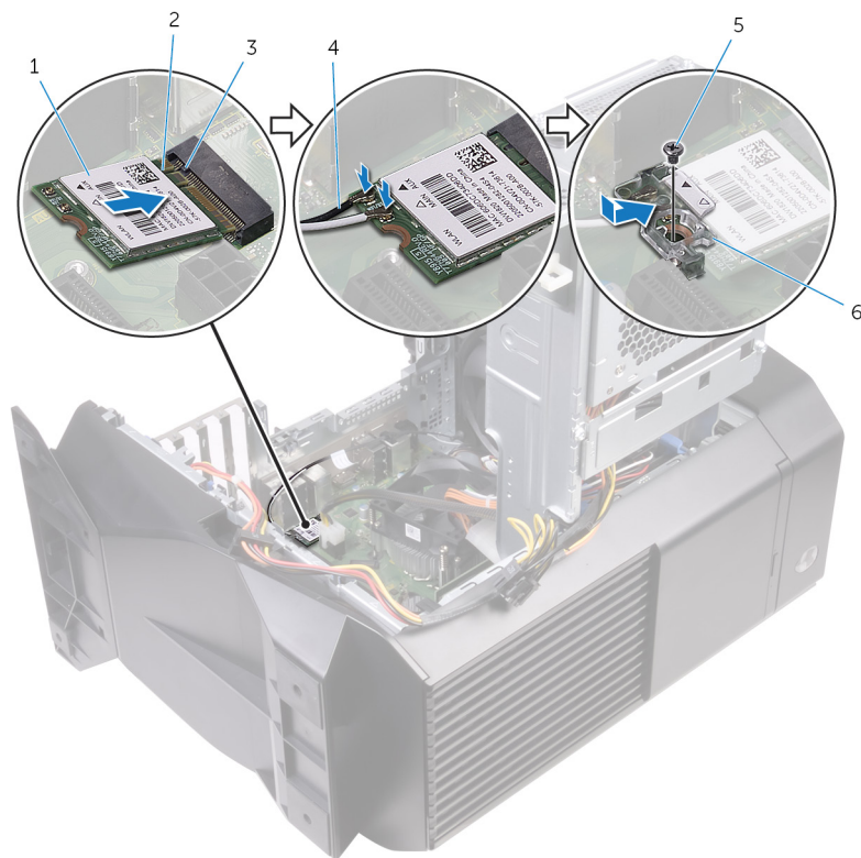
Abbildung 39. Wiedereinbauen der Wireless-Karte
