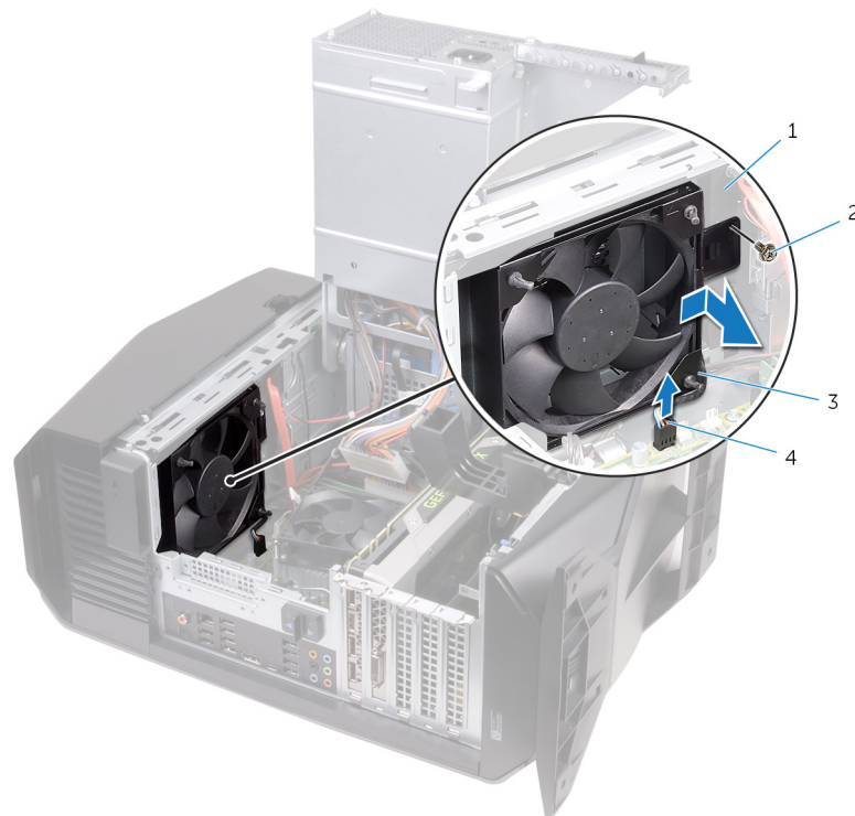
Figur 6. Ta bort den övre chassiflätten
