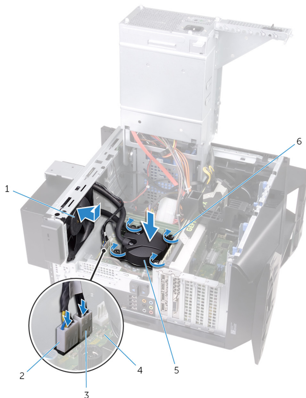
Figur 11. Sätta tillbaka processorns kylningsenhet
