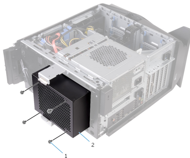
Figur 13. Sådan genmonteres processorkølemodulet
