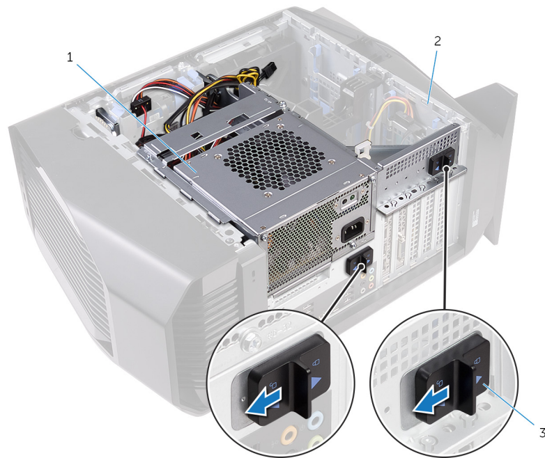
Figur 2. Sådan skubbes udløserlåsene for strømforsyningsenhedens kabinet
