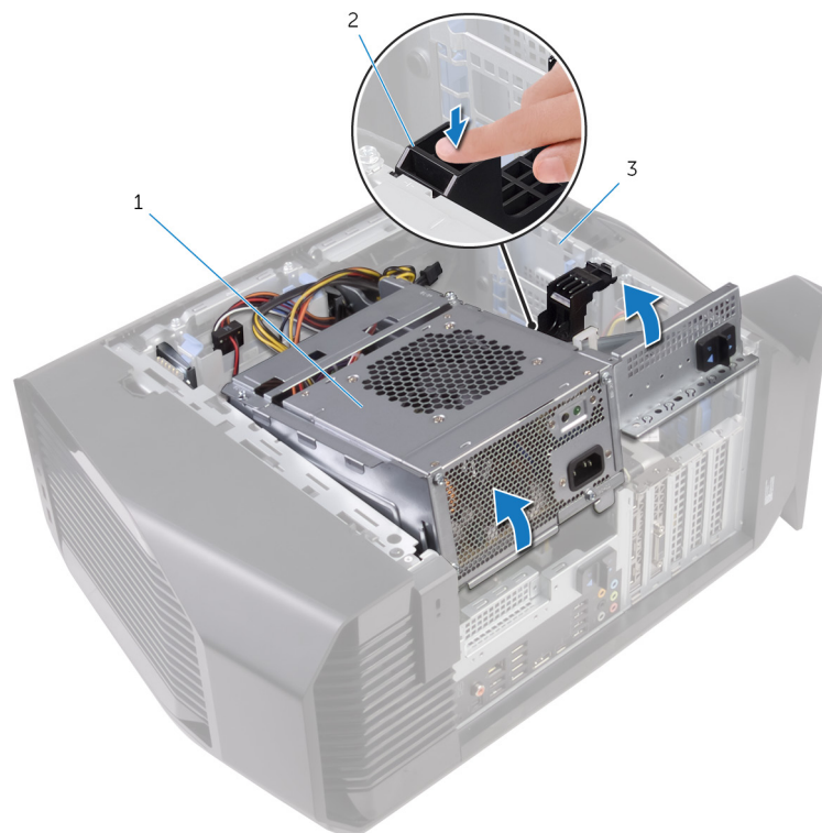
Figur 3. Sådan roteres strømforsyningsenheden
