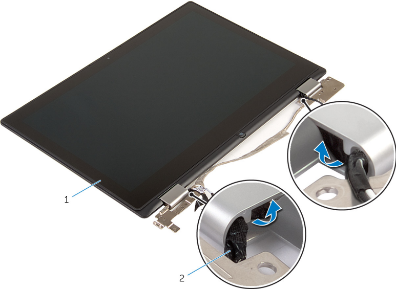
1 顯示板組件
