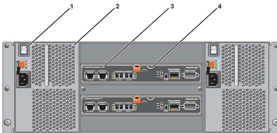
Ilustración 7: Componentes del panel posterior (4U)
