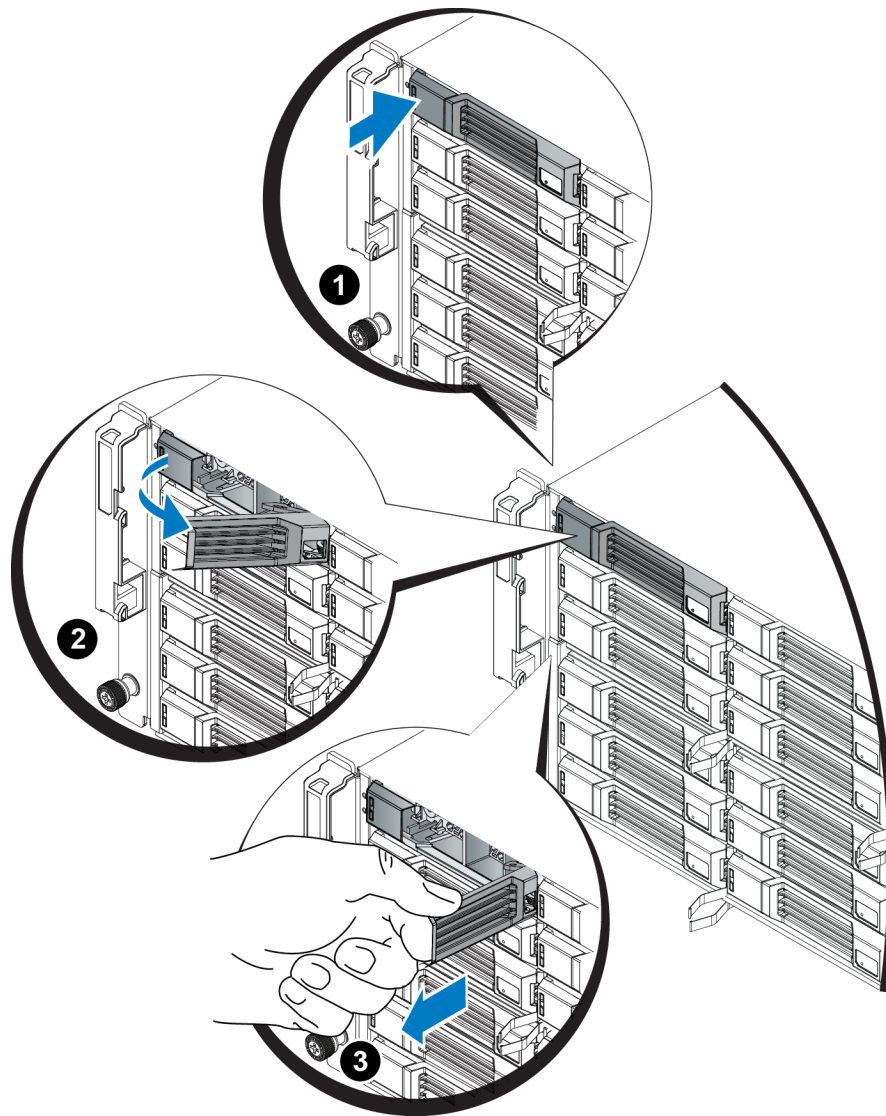
Ilustración 12: Extracción de una unidad de 3,5 pulgadas
