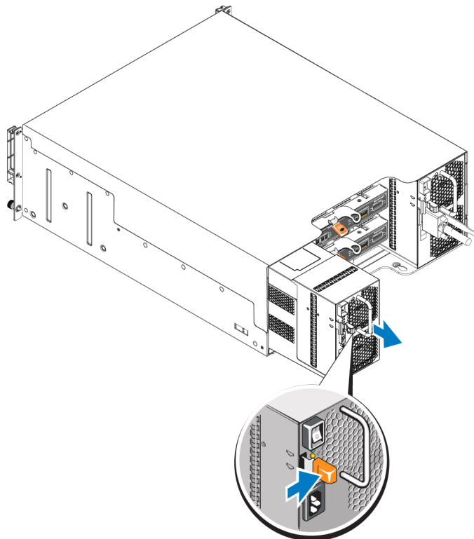
Ilustración 31: Extracción de un módulo de refrigeración y de un suministro de alimentación de 1080 W
