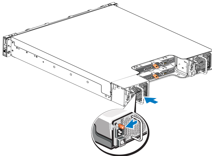
Ilustración 33: Introducción de un módulo de refrigeración y de un suministro de alimentación de 1080 W
