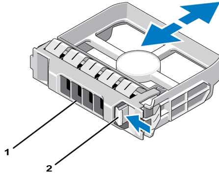
Ilustración 15: Extracción e instalación de una unidad de disco duro de relleno de 2,5 pulgadas.
