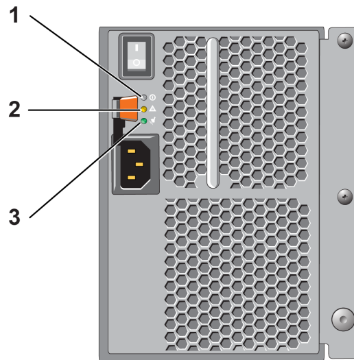
Ilustración 29: LED del suministro de alimentación de 1080 W (arreglos 4U)
