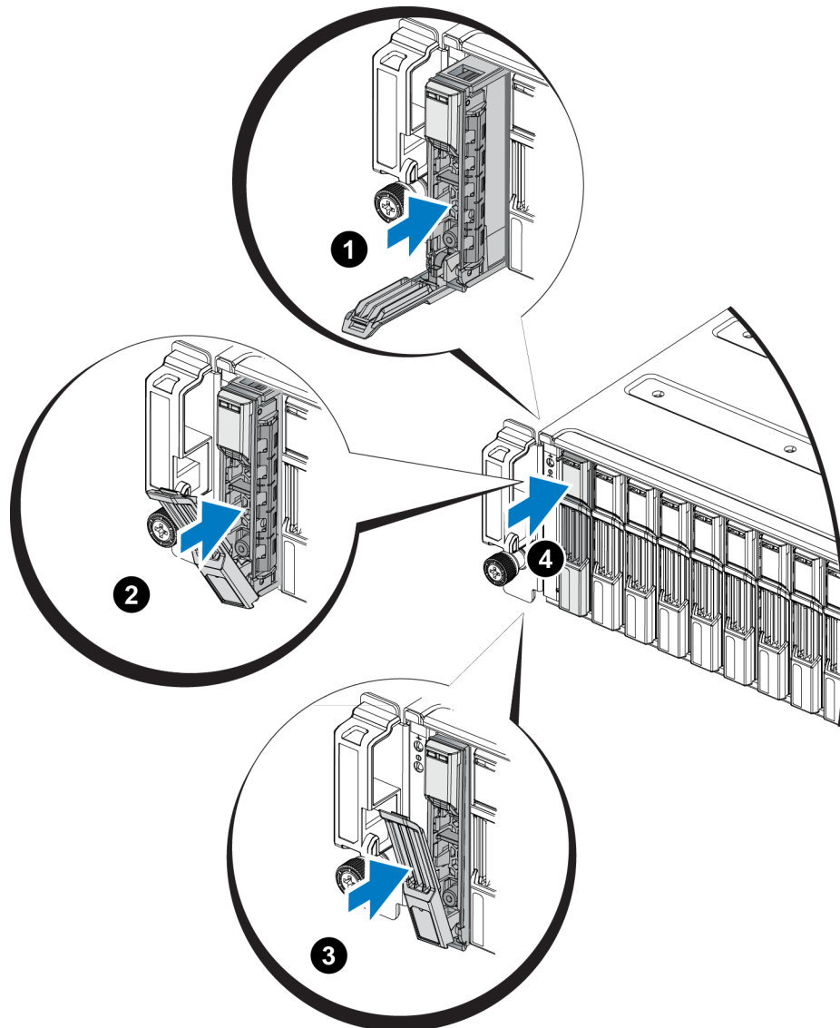
Ilustración 11: Instalación de una unidad de 2,5 pulgadas
