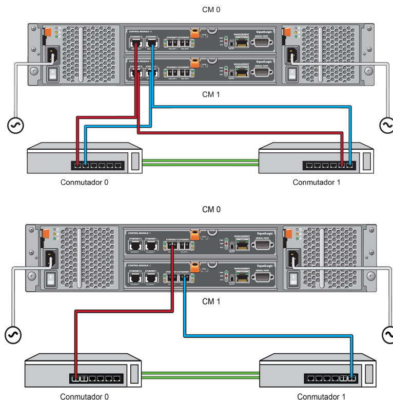
Ilustración 16: Configuración de red recomendada para admitir la conmutación por error vertical
