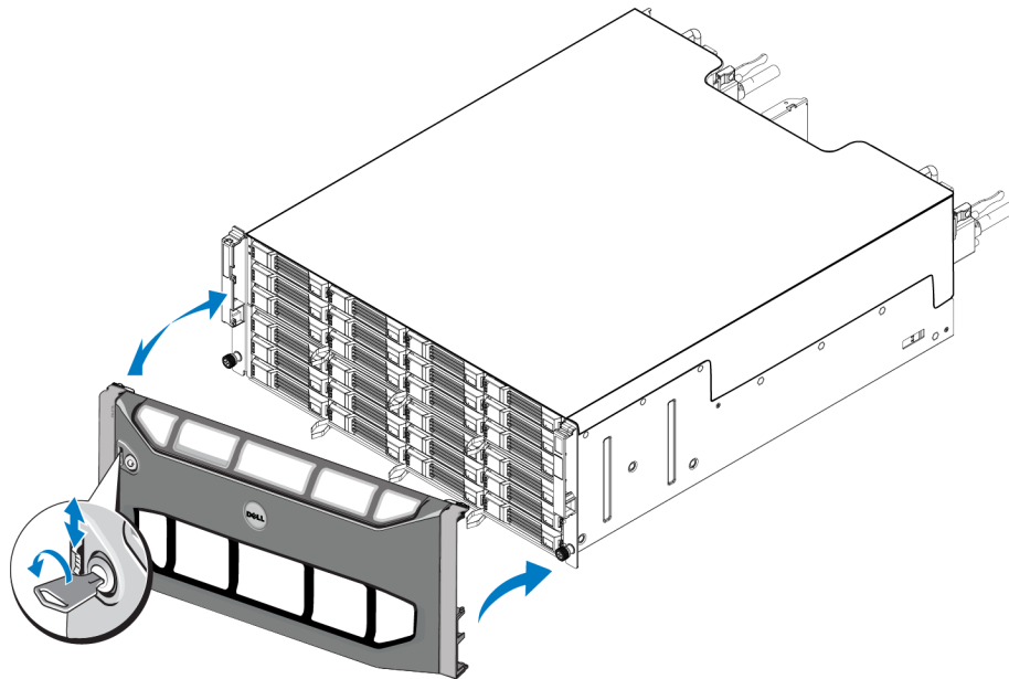
Ilustración 3: Instalación del bisel (arreglo 4U)
