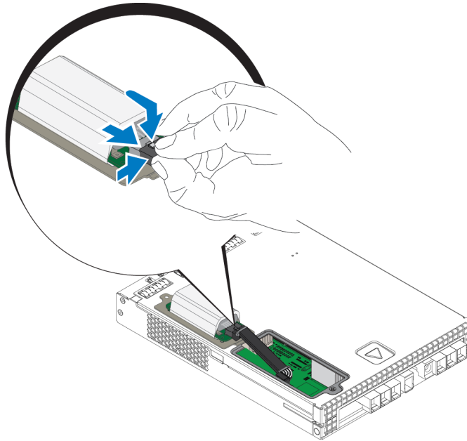
Ilustración 26: Desconexión de la batería
