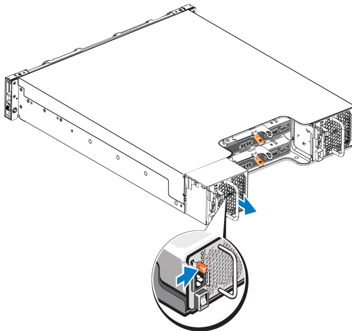
Ilustración 30: Extracción de un módulo de refrigeración y de un suministro de alimentación de 700 W
