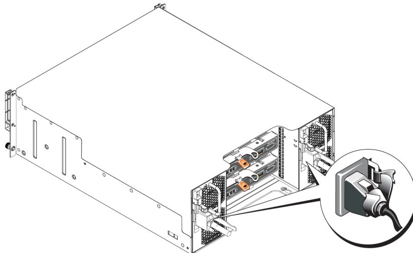
Ilustración 35: Fijación de los cables de alimentación (suministro de alimentación de 1080 W)
