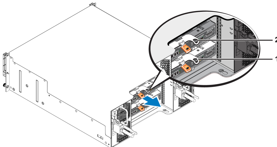
Ilustración 19: Extracción de un módulo de control (arreglo 4U)
