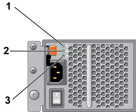
Ilustración 28: LED del suministro de alimentación de 700 W (arreglos 2U)
