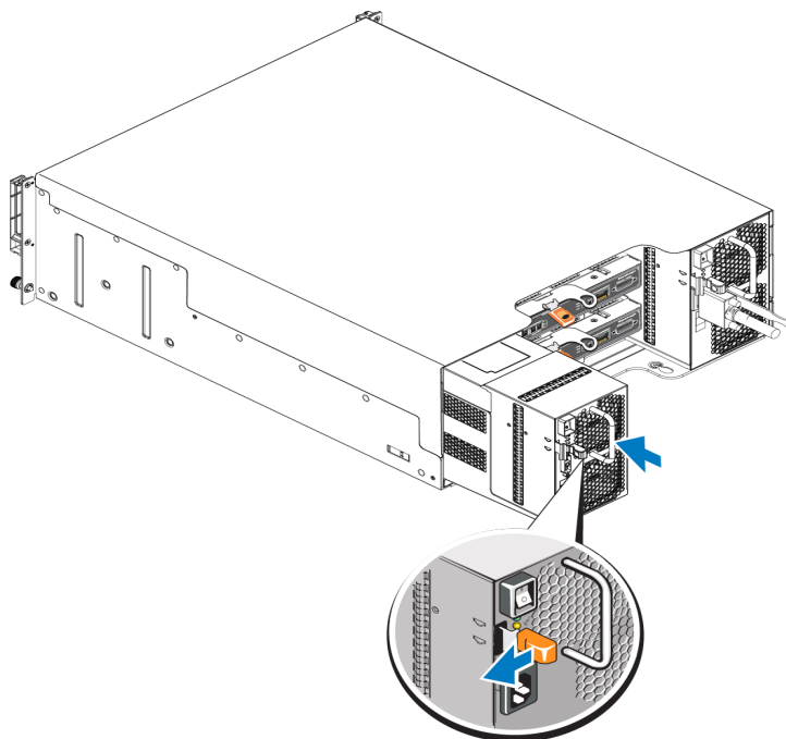
Ilustración 33: Introducción de un módulo de refrigeración y de un suministro de alimentación de 1080 W
