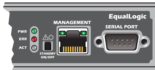
Ilustración 18: Ubicación del botón del modo en espera
