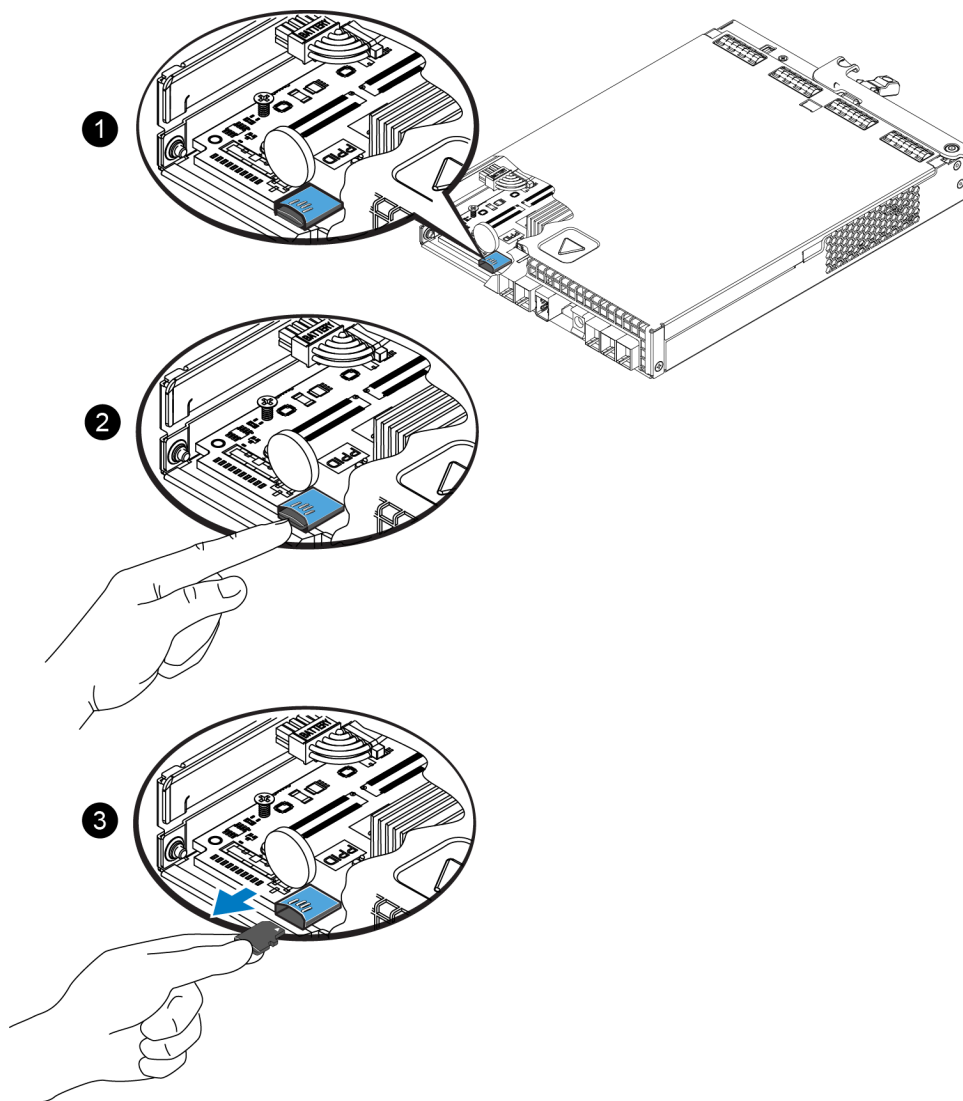
Ilustración 22: Expulsión de la tarjeta microSD
