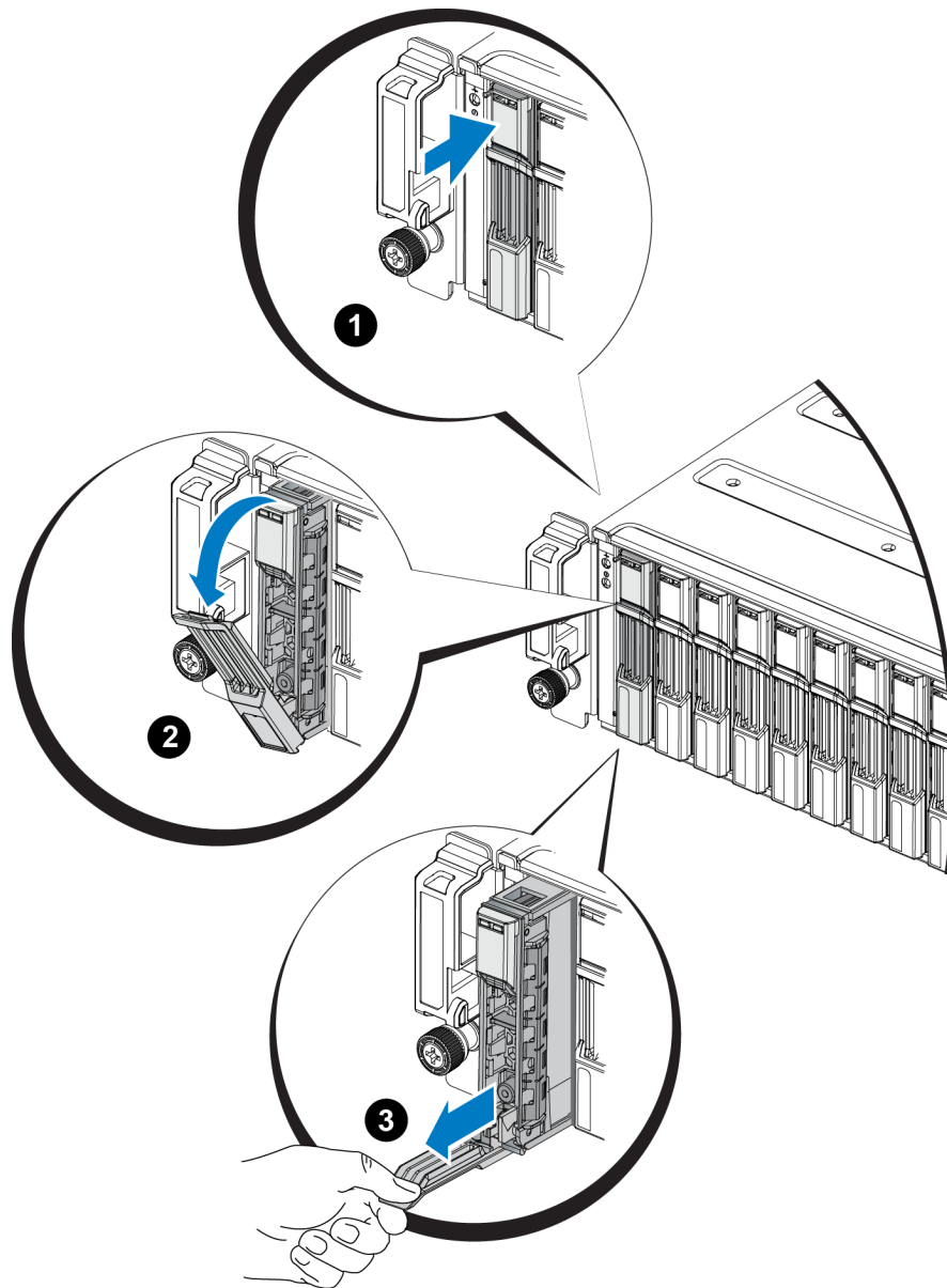
Ilustración 10: Extracción de una unidad de 2,5 pulgadas
