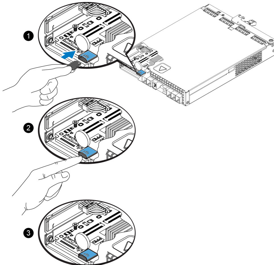
Ilustración 23: Inserción de la tarjeta MicroSD
