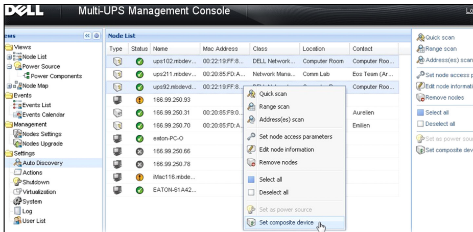
Рис. 82. Выбор композиционного устройства узла для настройки
