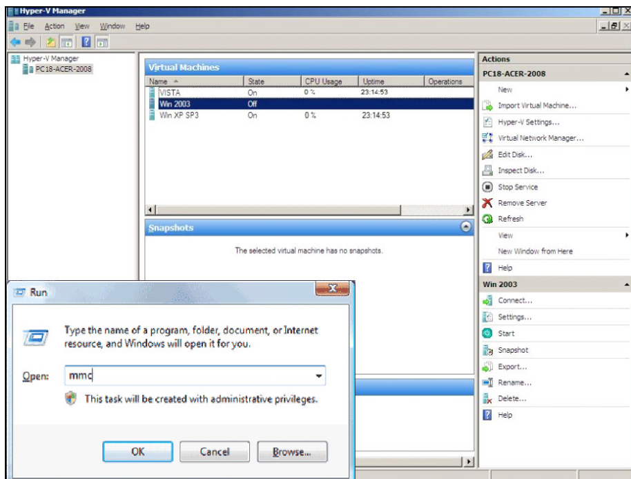
図 76.Hyper-V マネージャ
