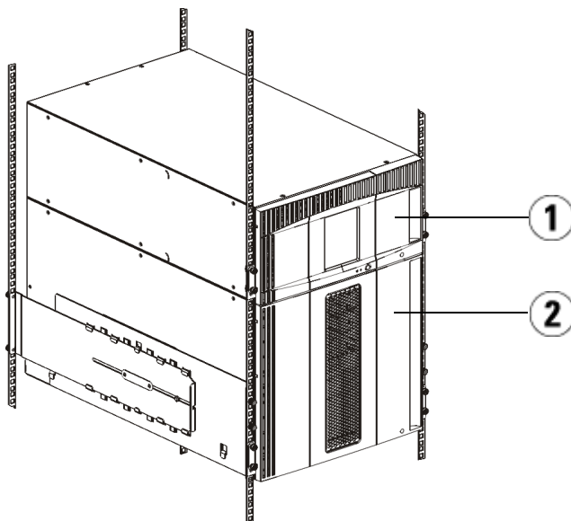
1 Módulo de controle de biblioteca de 5U 2 Módulo de expansão de biblioteca de 9U
