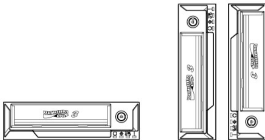
Рис. 3. Допустимые ориентации при монтаже
