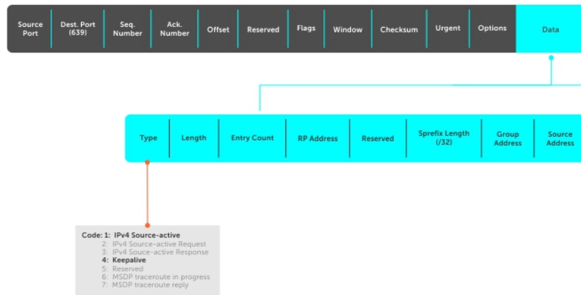
Figure 73. MSDP SA Message Format
