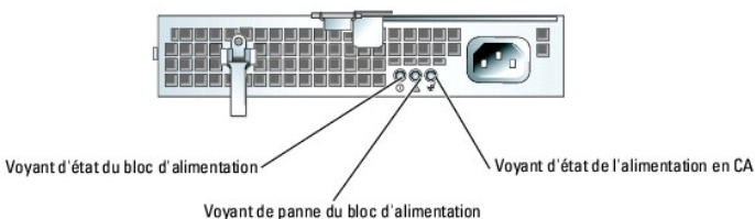
Figure 1-4. Voyants des blocs d'alimentation redondants
