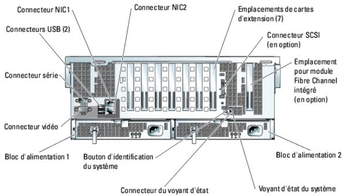
Figure 1-3. Caractéristiques et voyants du panneau arrière
