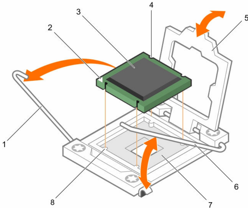
图 40: 安装和卸下处理器
