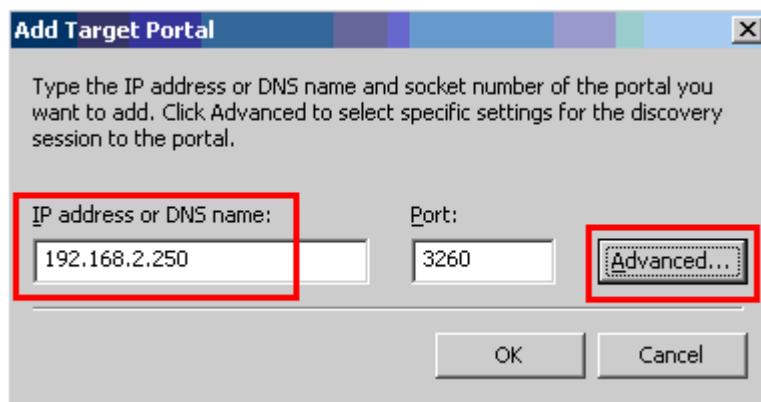
图 10-9. “添加目标门户”对话框
