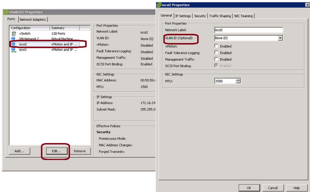
图 8-2. VM 网络属性：实例 2
