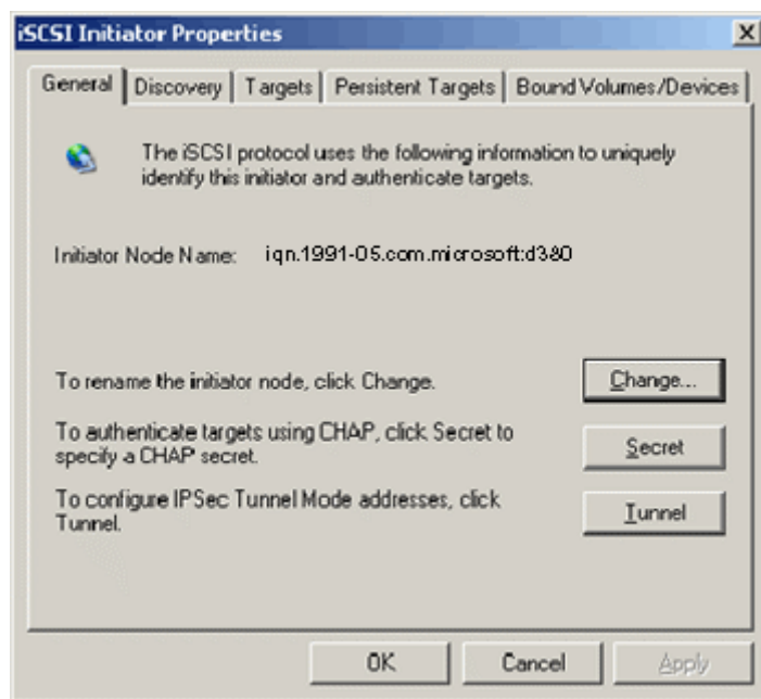
图 10-6. “iSCSI 启动器属性”：“常规”页面
