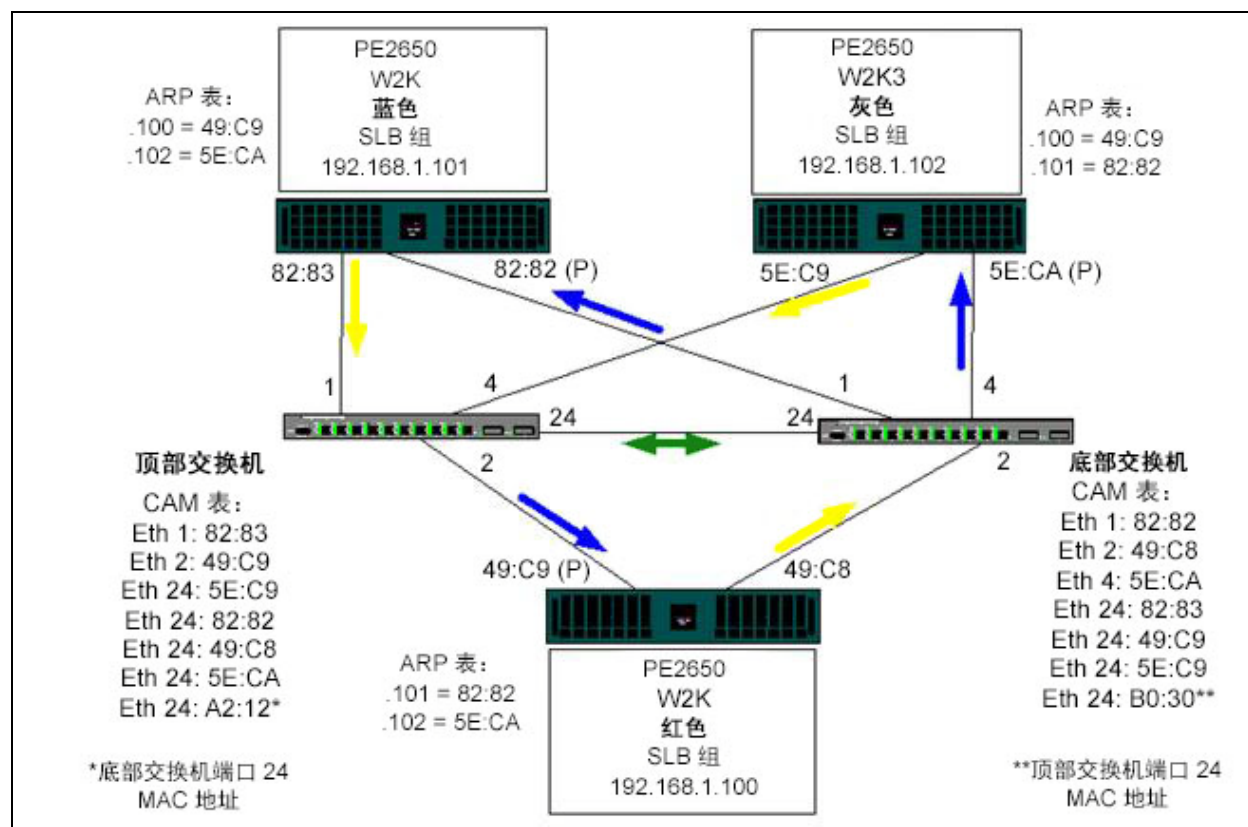
图 11-4. 有互连的跨交换机组合
