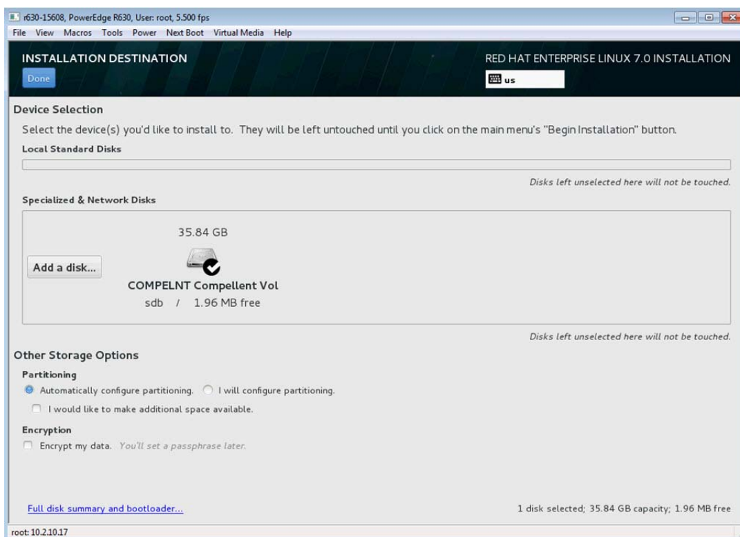
图 14-30. 选择分区选项
