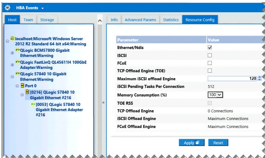
图 14-39. 资源配置页面
