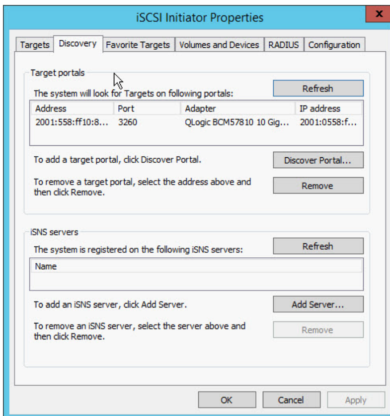
图 10-11. “iSCSI 启动器属性”：“发现”页面
