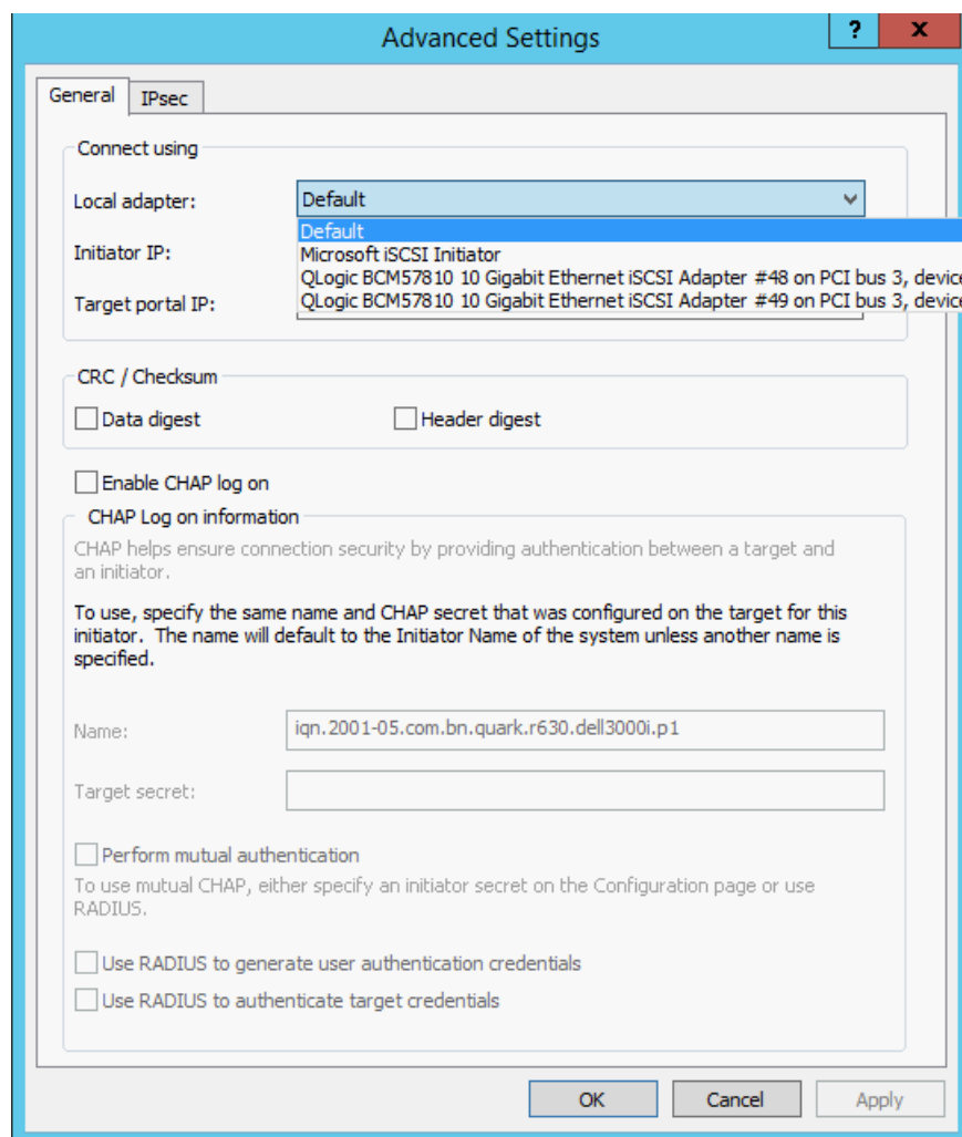
图 10-14. “高级设置”：“常规”页面，“本地适配器”
