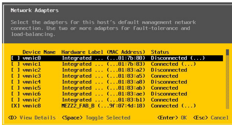
图 14-35. ESXi 管理网络选择
