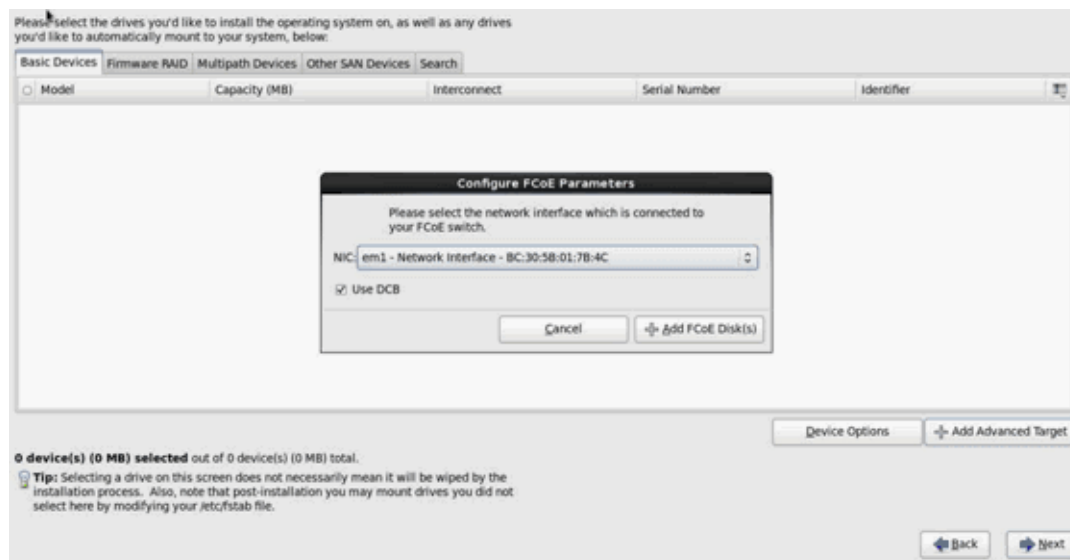
图 14-27. 配置 FCoE 参数
