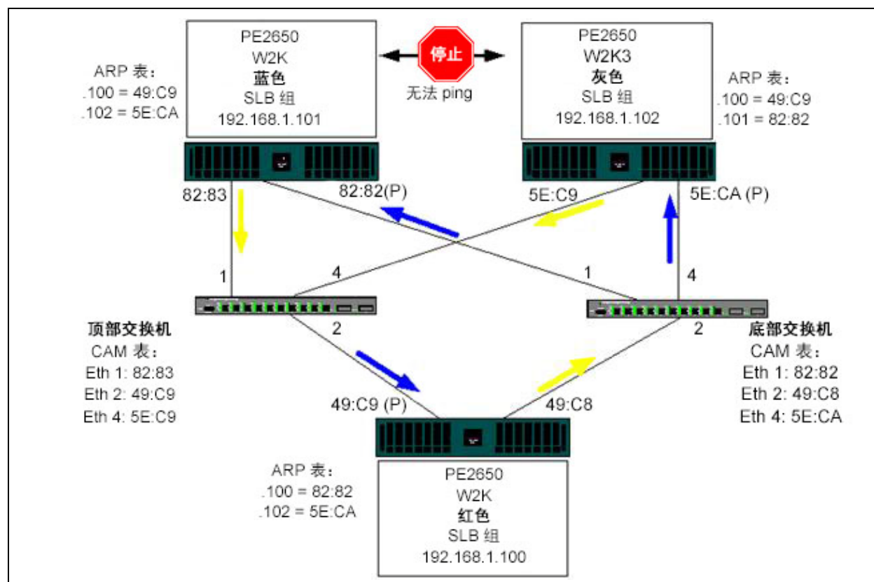
图 11-3. 无交换机间链路的跨交换机组合
