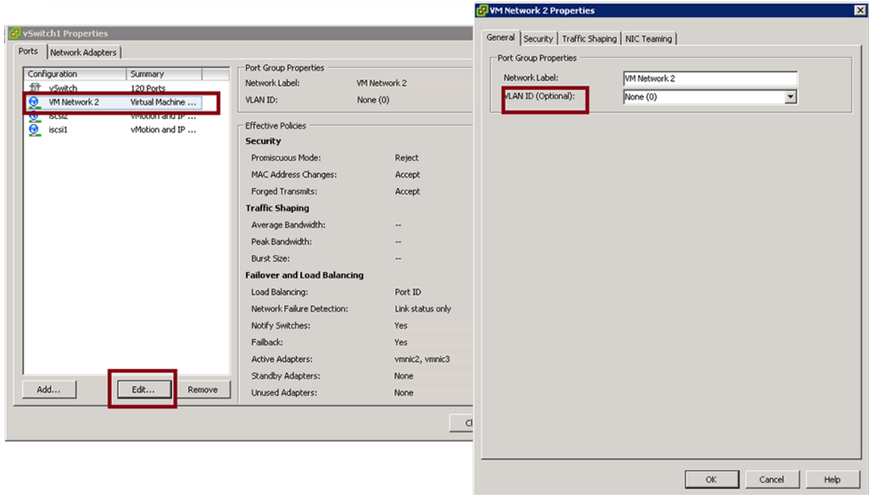
图 8-1. VM 网络属性: 实例 1
