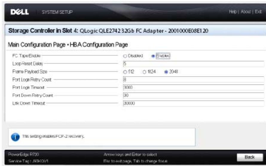
그림 3-16. Dell 시스템 설정 : HBA 구성
