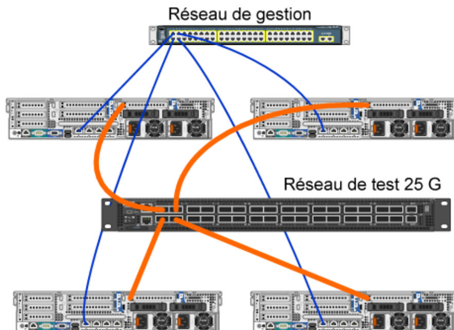
Figure 13-18. Exemple de configuration matérielle
