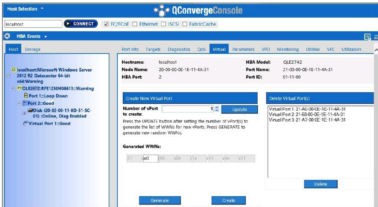
Figura 3-35. Criação de uma porta virtual
