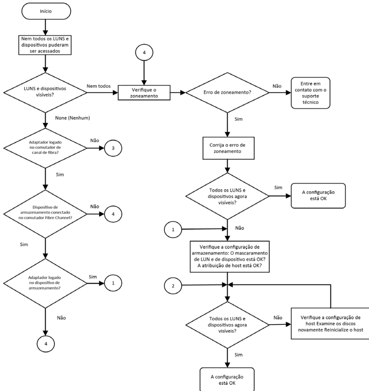
Figura A-1. Diagrama de solução de problemas de fibre channel (1 de 2)
