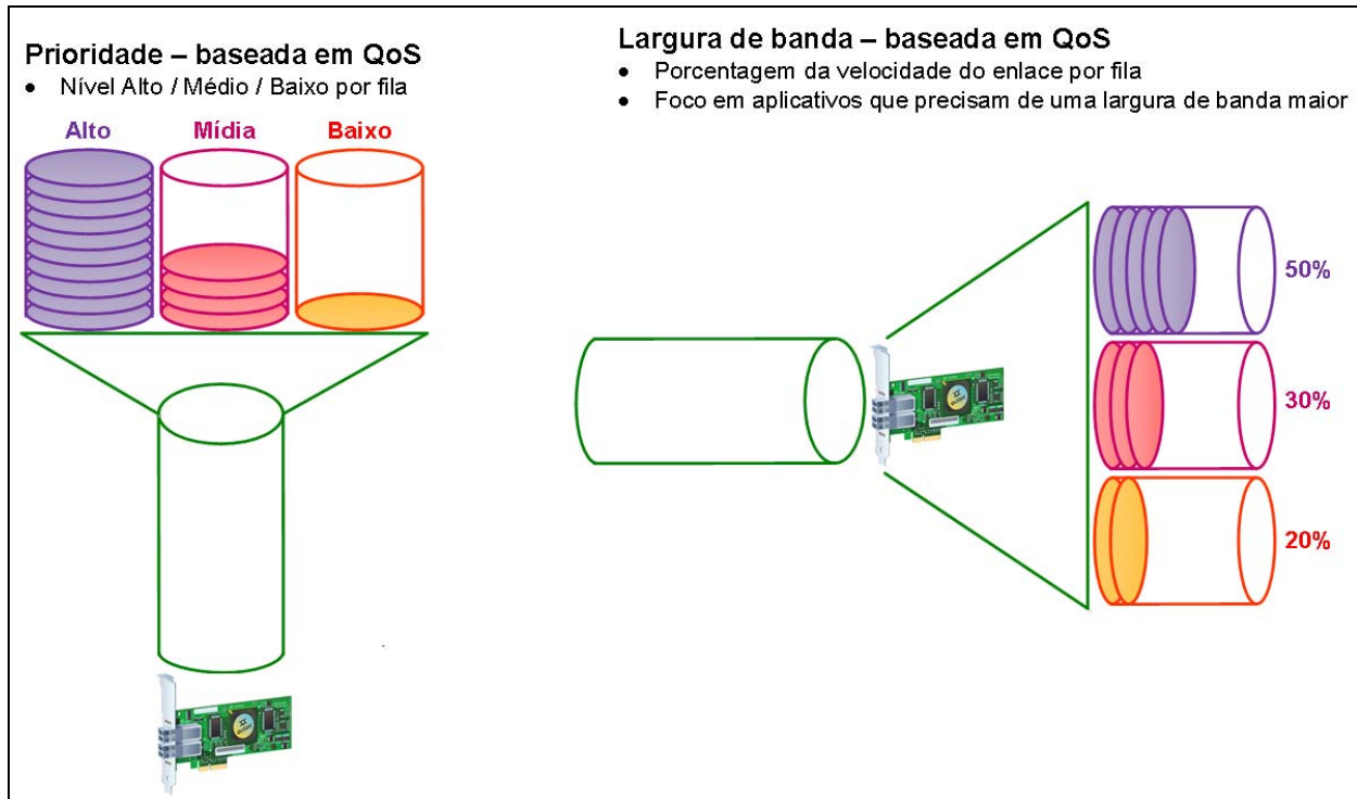
Figura 3-7. QoS baseada em prioridade e em largura de banda
