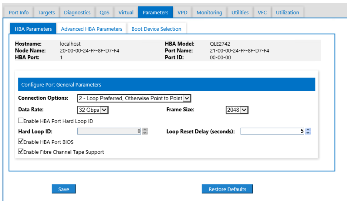
Figura 3-23. Habilitar o BIOS da porta do adaptador de barramento de host
