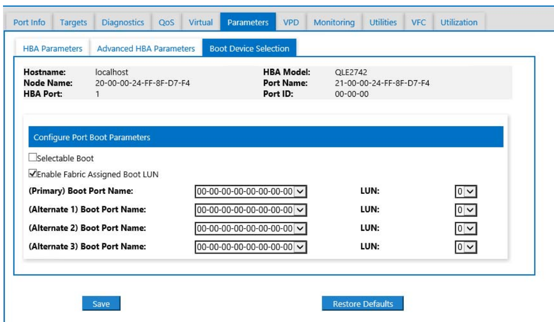
Figura 3-24. Habilitar LUN de inicialização atribuído à malha
