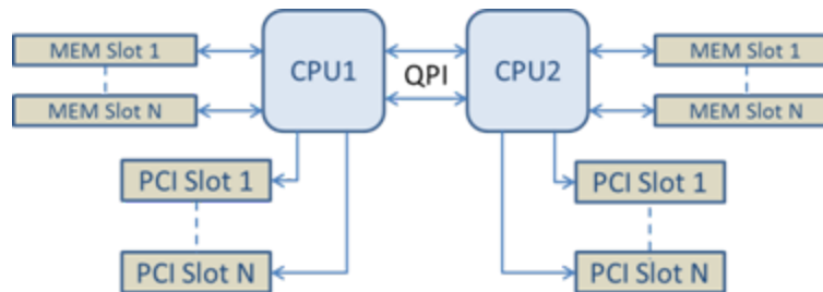
Arquitetura de memória / PCI de raiz múltipla distribuída
