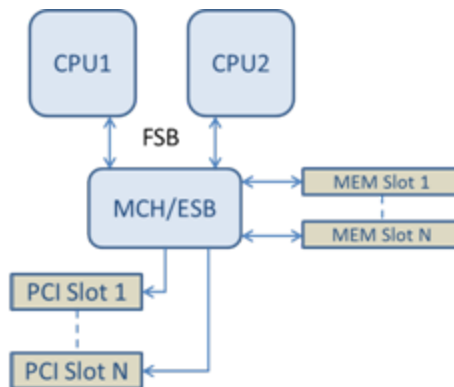
Arquitectura de memoria/PCI de raíz única compartida
