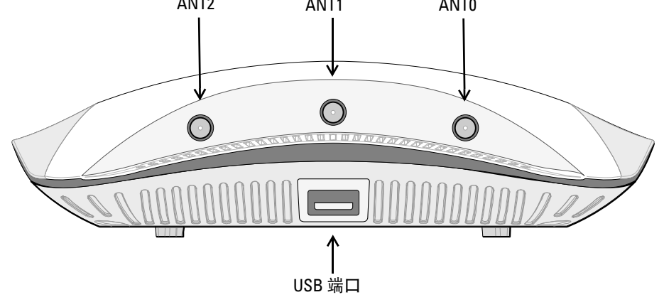
图 2 W-AP210 系列侧视图 (W-AP214 显示)
