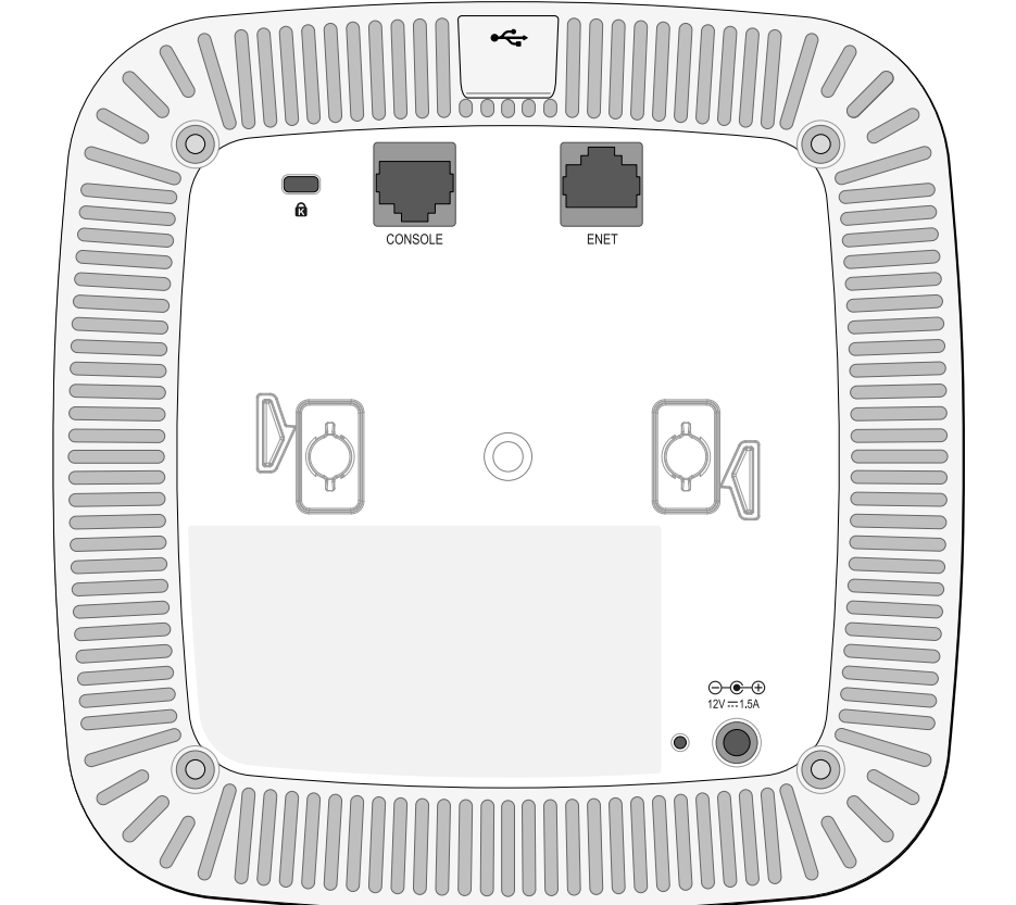
图 4 W-AP210 系列底视图
