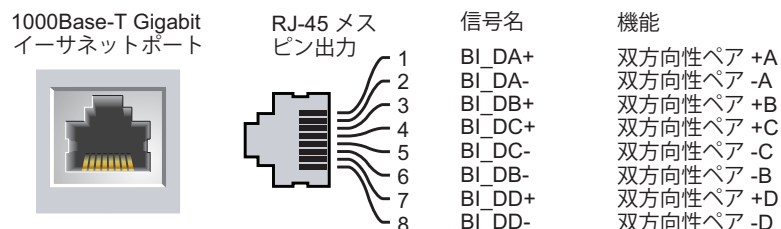
図 3 Gigabit イーサネットポートピン出力
