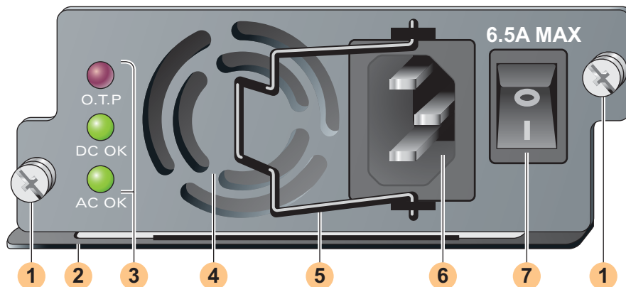
Figura 1 Fonte de alimentação de 400 W
