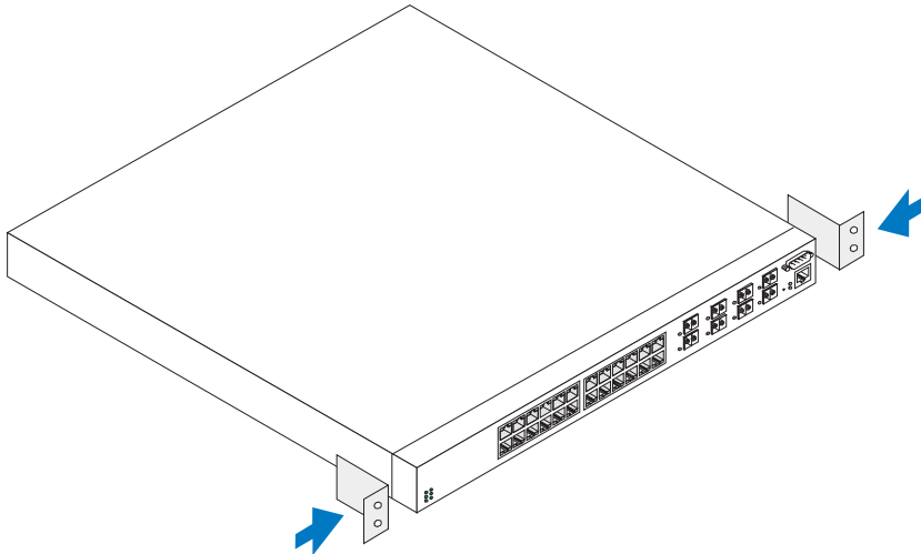
图 1-1. 连接支架
