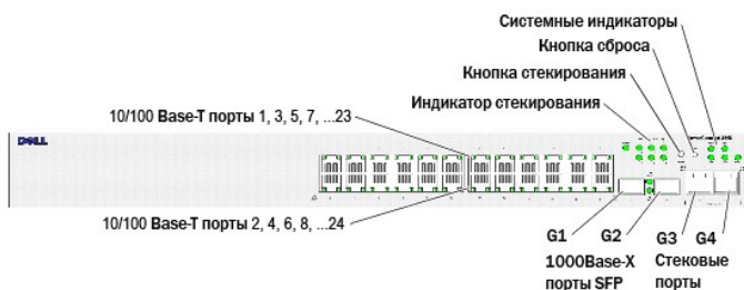
Рис 2-1. Передняя панель устройства PowerConnect 3524
