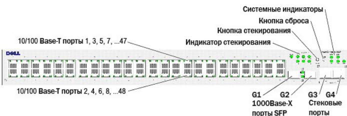
Рис 2-3. Передняя панель устройства PowerConnect 3548
