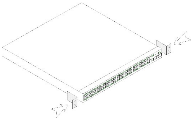
Рис. 3-1. Установка монтажного кронштейна и крепление устройства на стойке
