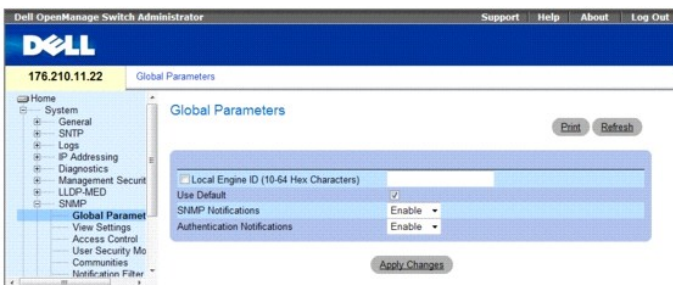
Рис. 6-87. Общие параметры SNMP
