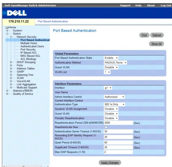
Рис. 7-1. Страница Port Based Authentication (Проверка подлинности на основе порта)
