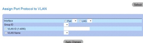
Рис. 7-58. Назначение порта протокола сети VLAN
