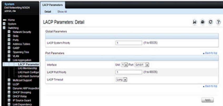
Figure 26-3. LACP Parameters
